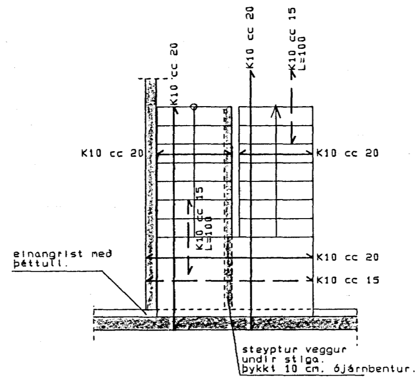
Járnending stiga. MKV 1:50
