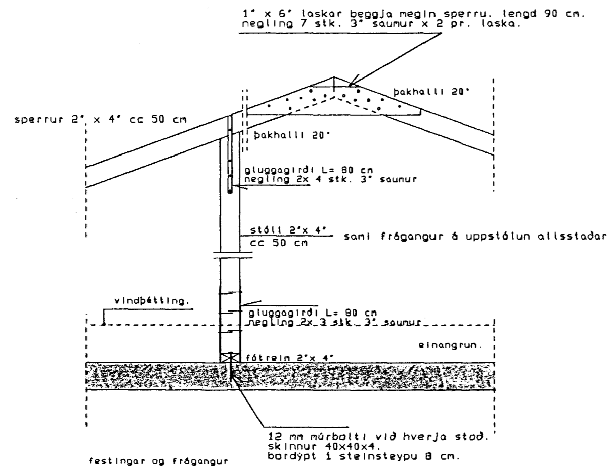
festingar og frágangur á sperrum í þakrymi. lóðrétt snið í þakrymi
