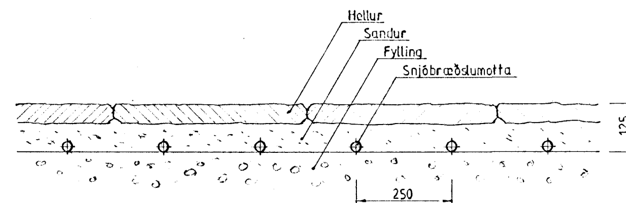
SNEIDING A-A
