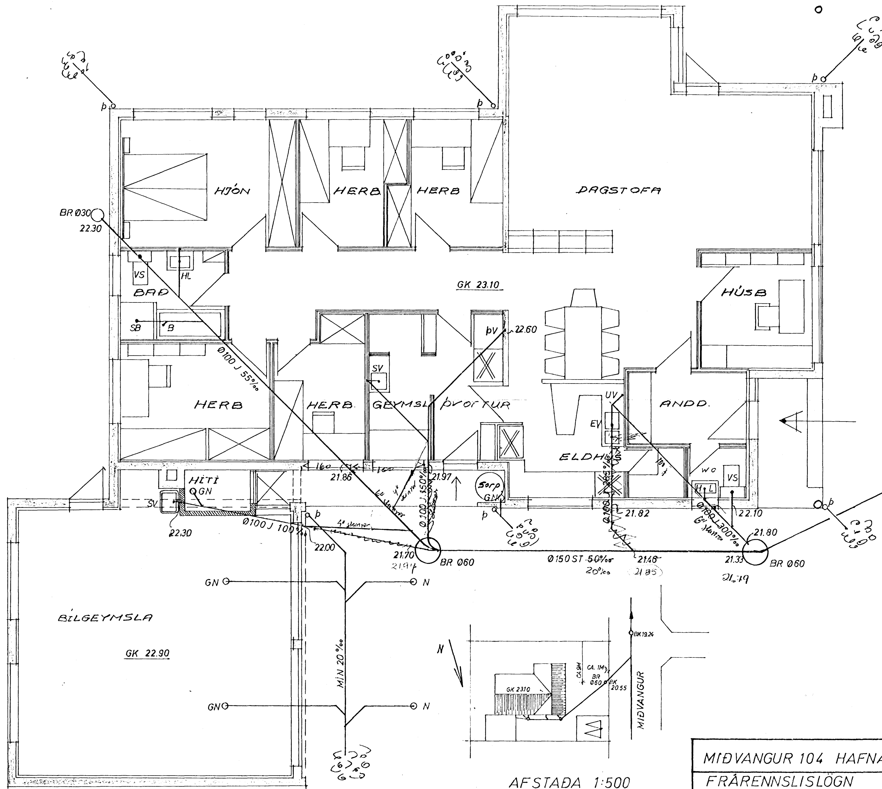
GRUNNMYND 1:50
