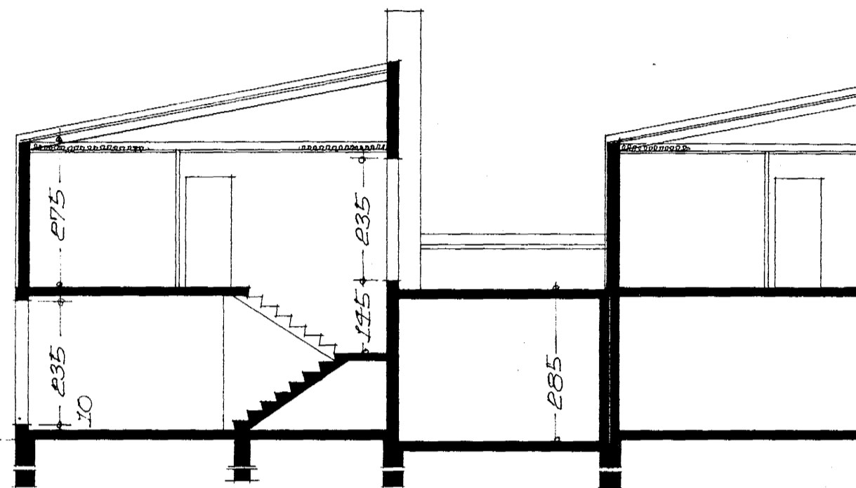
SKURÐUR B-B
