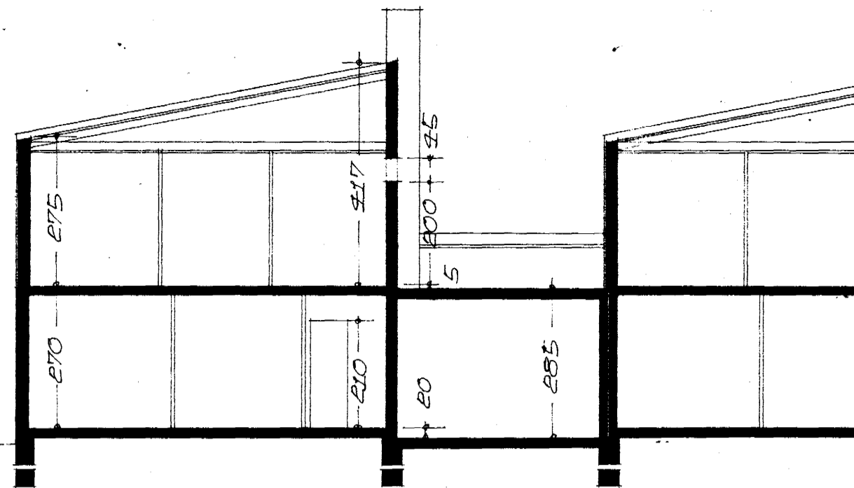
SKURÐUR A-A
