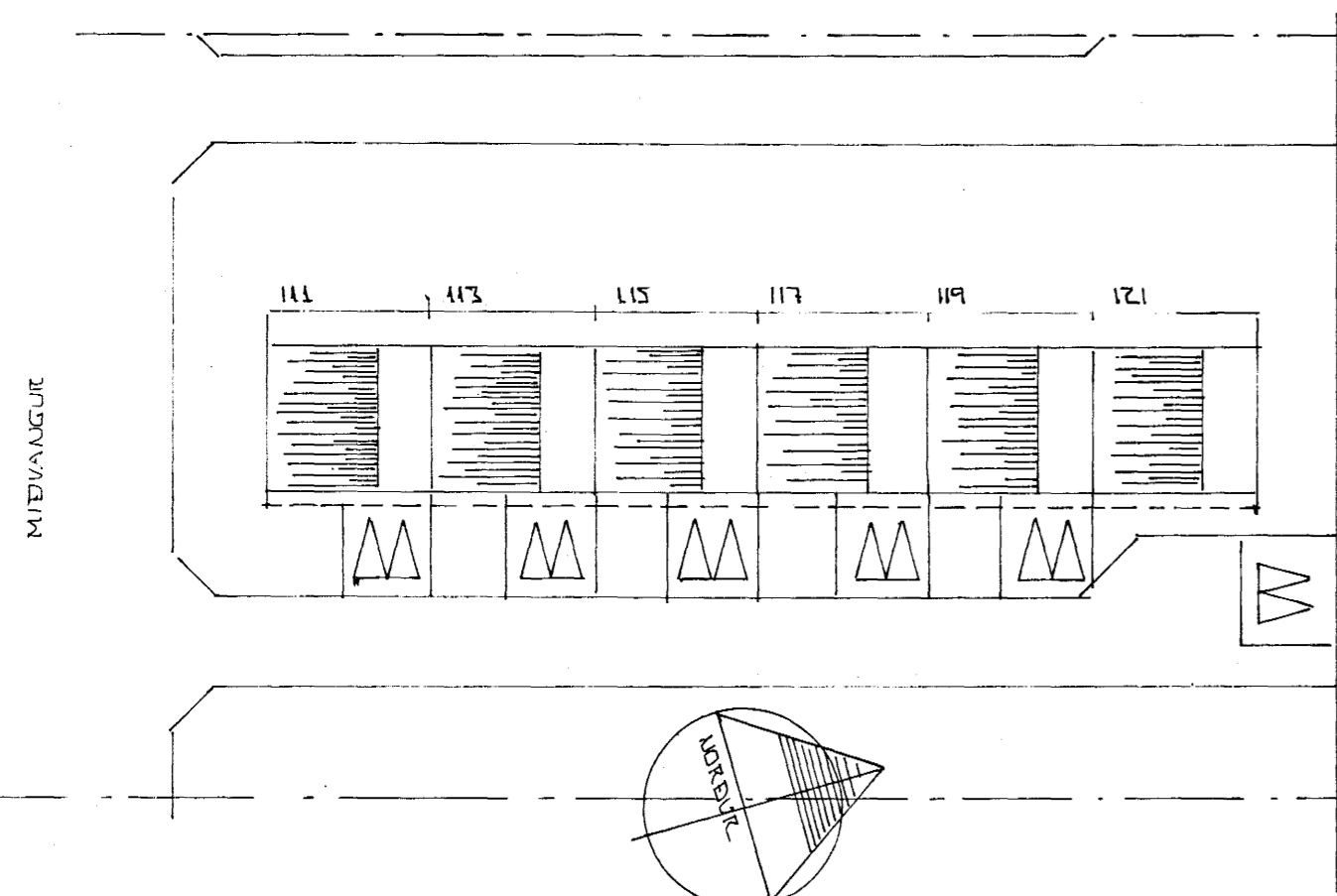
AFSTOÐUMYND 1:500
