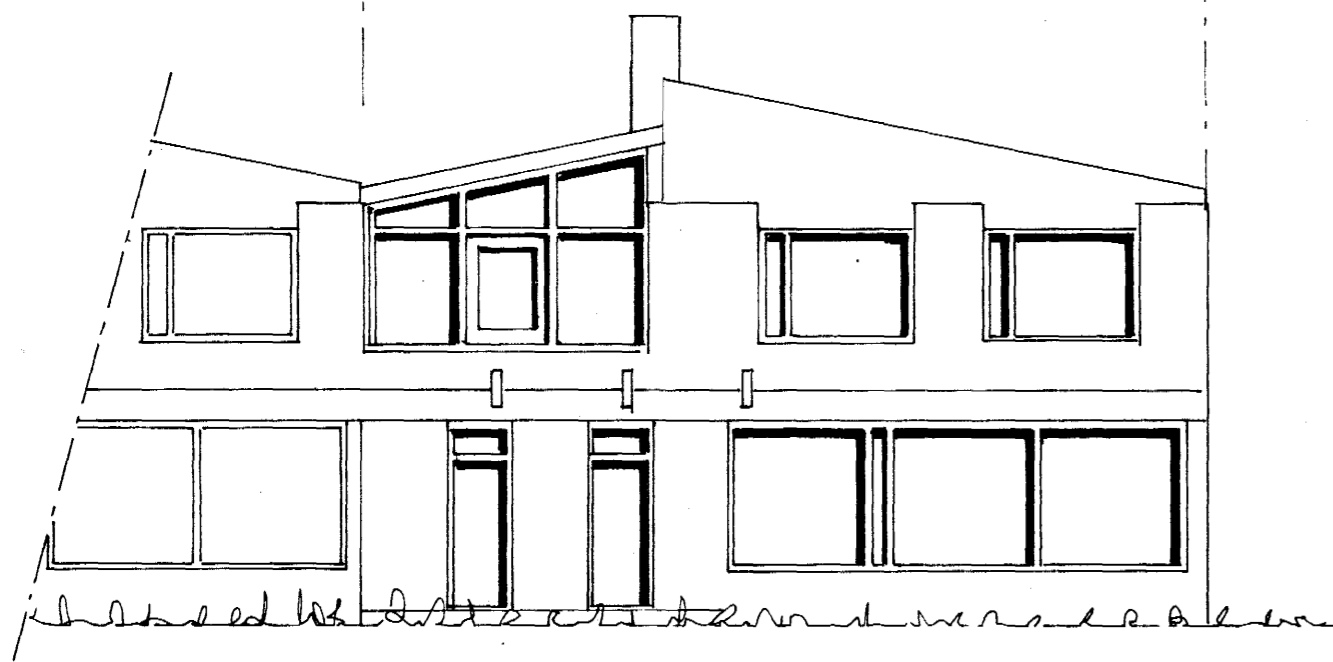
ÚTLIT VESTUR 1:100
