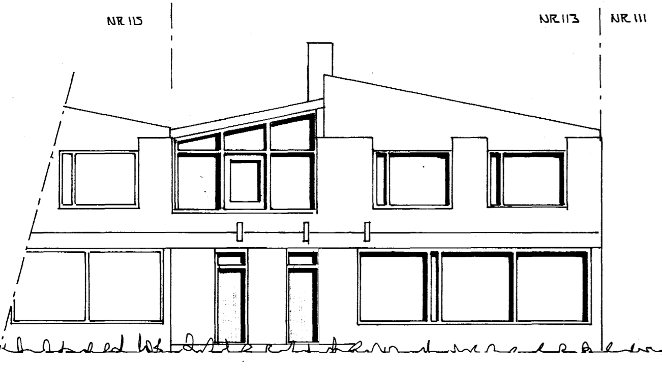
ÚTLIT VESTUR 1:100
