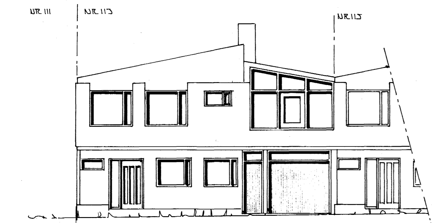
ÚTLIT AUSTUR 1:100
