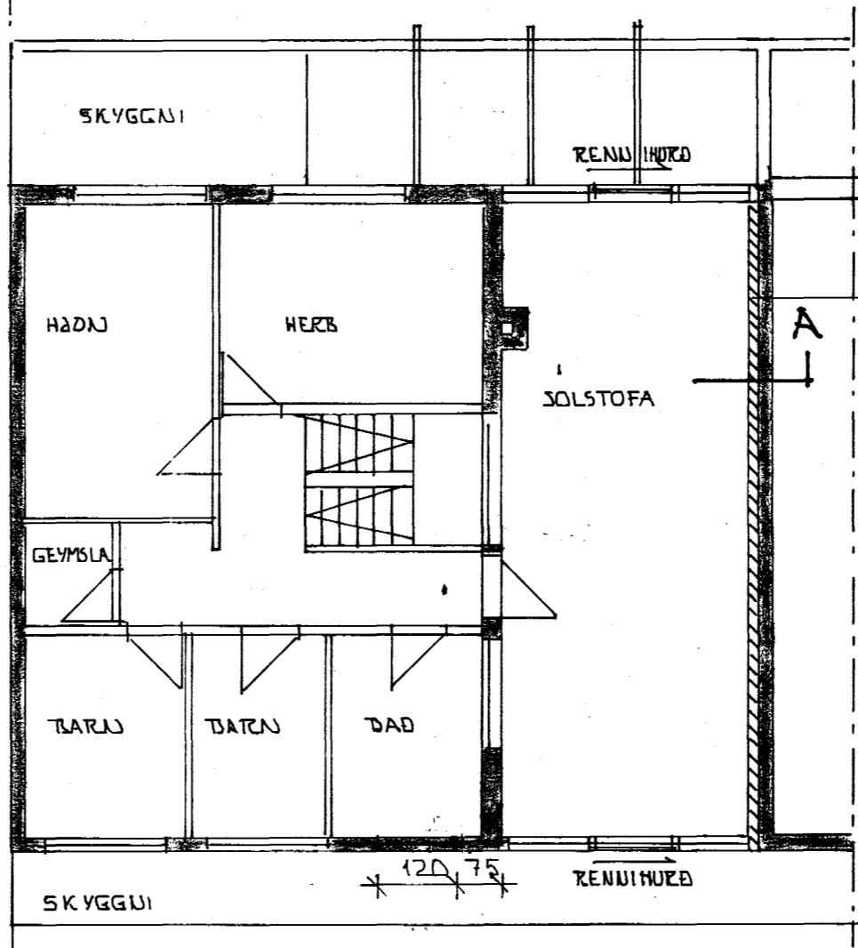
GRUNNMYND 1:100
