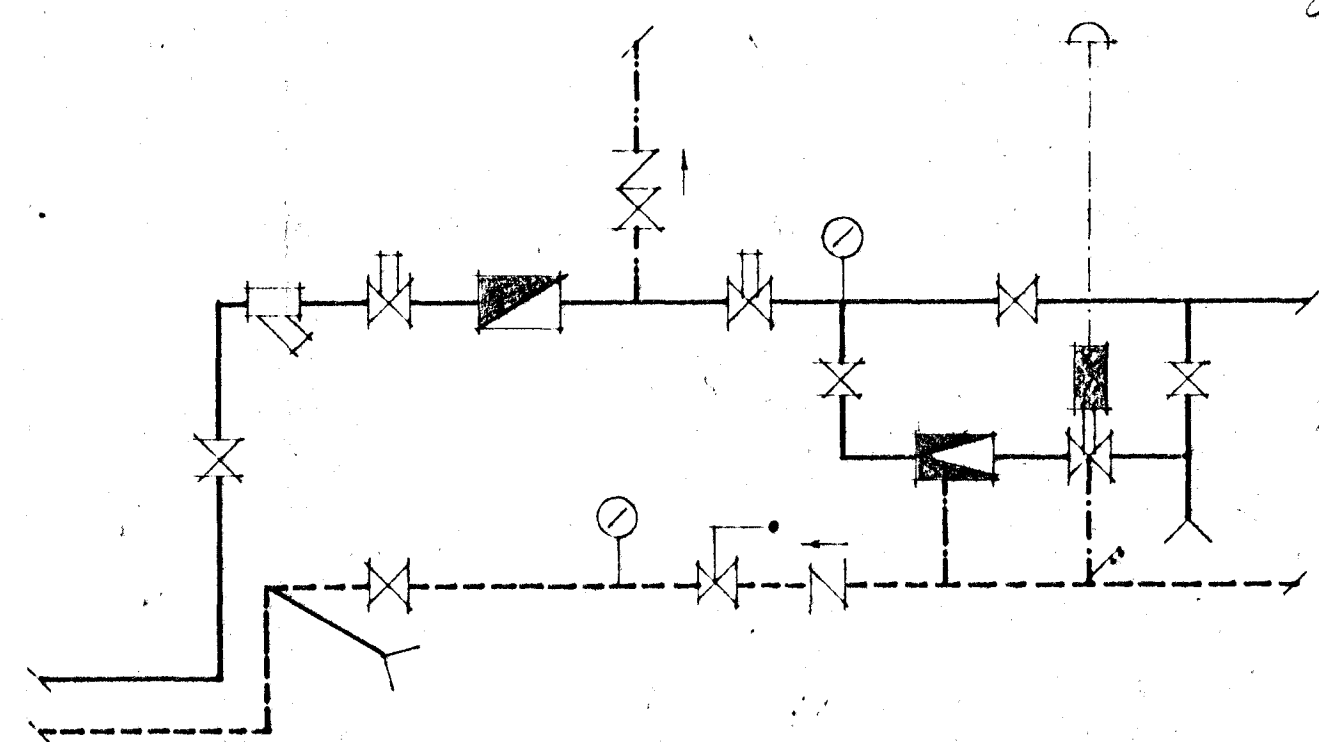
TENGING VIÐ HITAVEITU (TVÓFALT KERFI).
