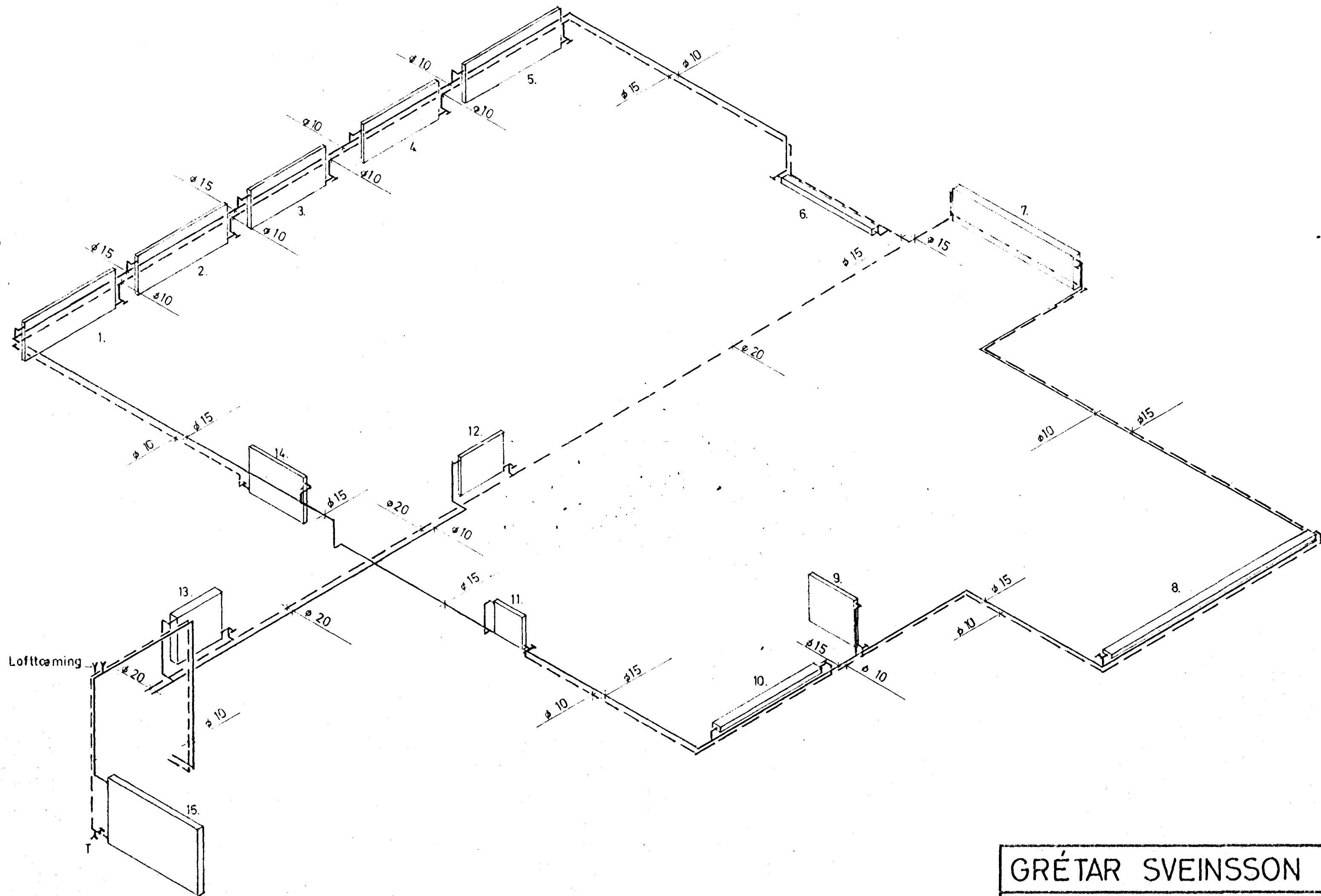
KERFISMYND 1:50
