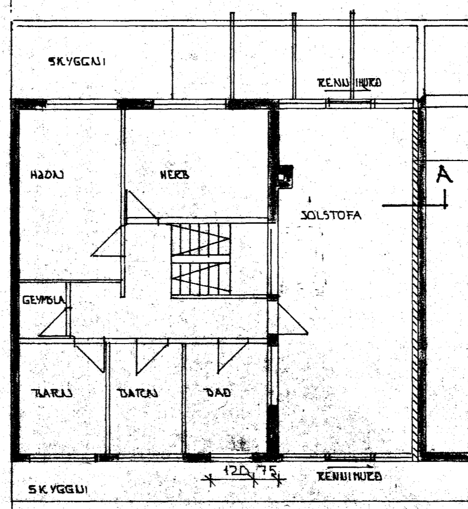
GRUNNMYND 1:100
