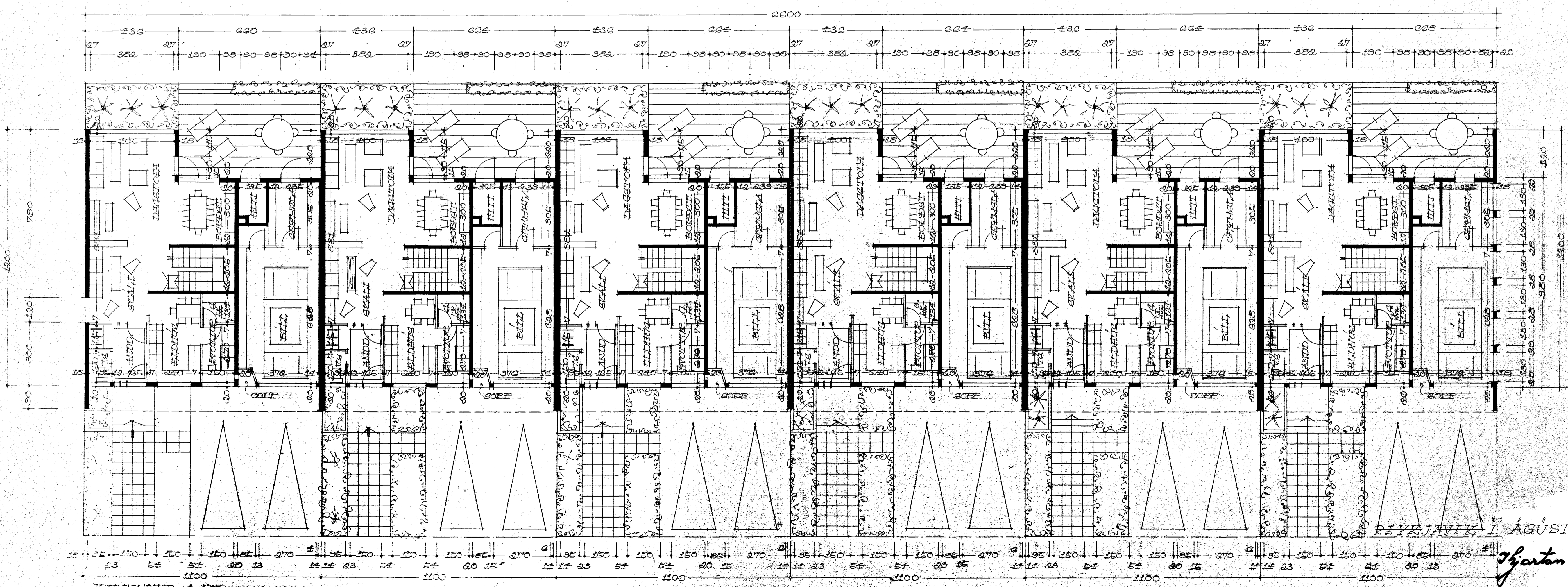
DRÖGNAFLUTRÚNN 2. HÆÐ
