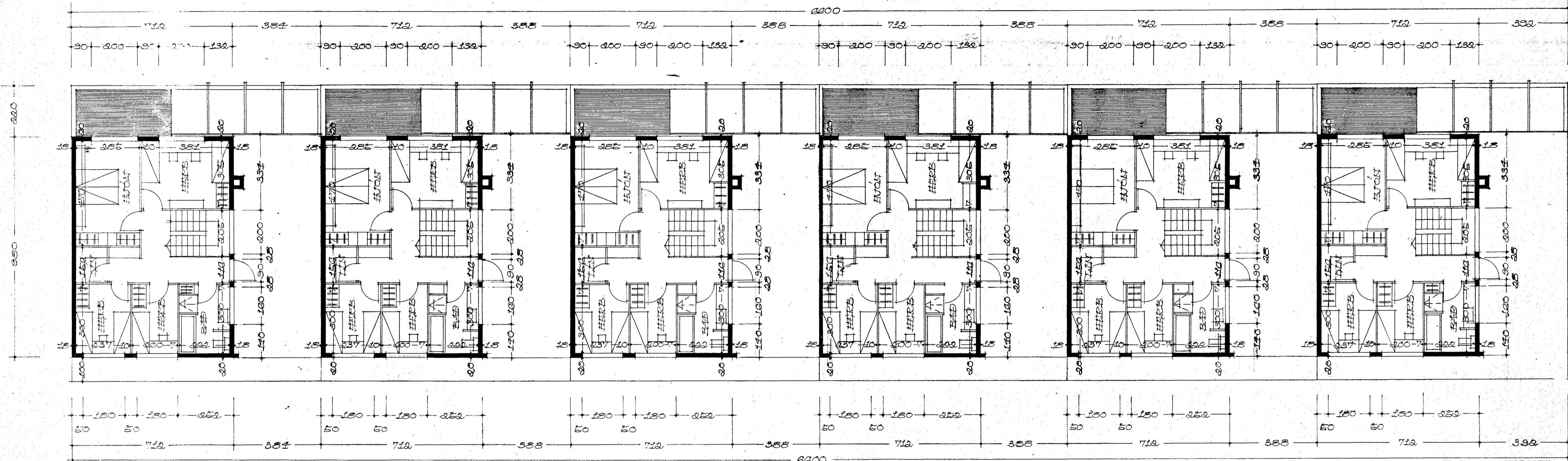
DRÖGNAFLUTRÚNN 1. HÆÐ
