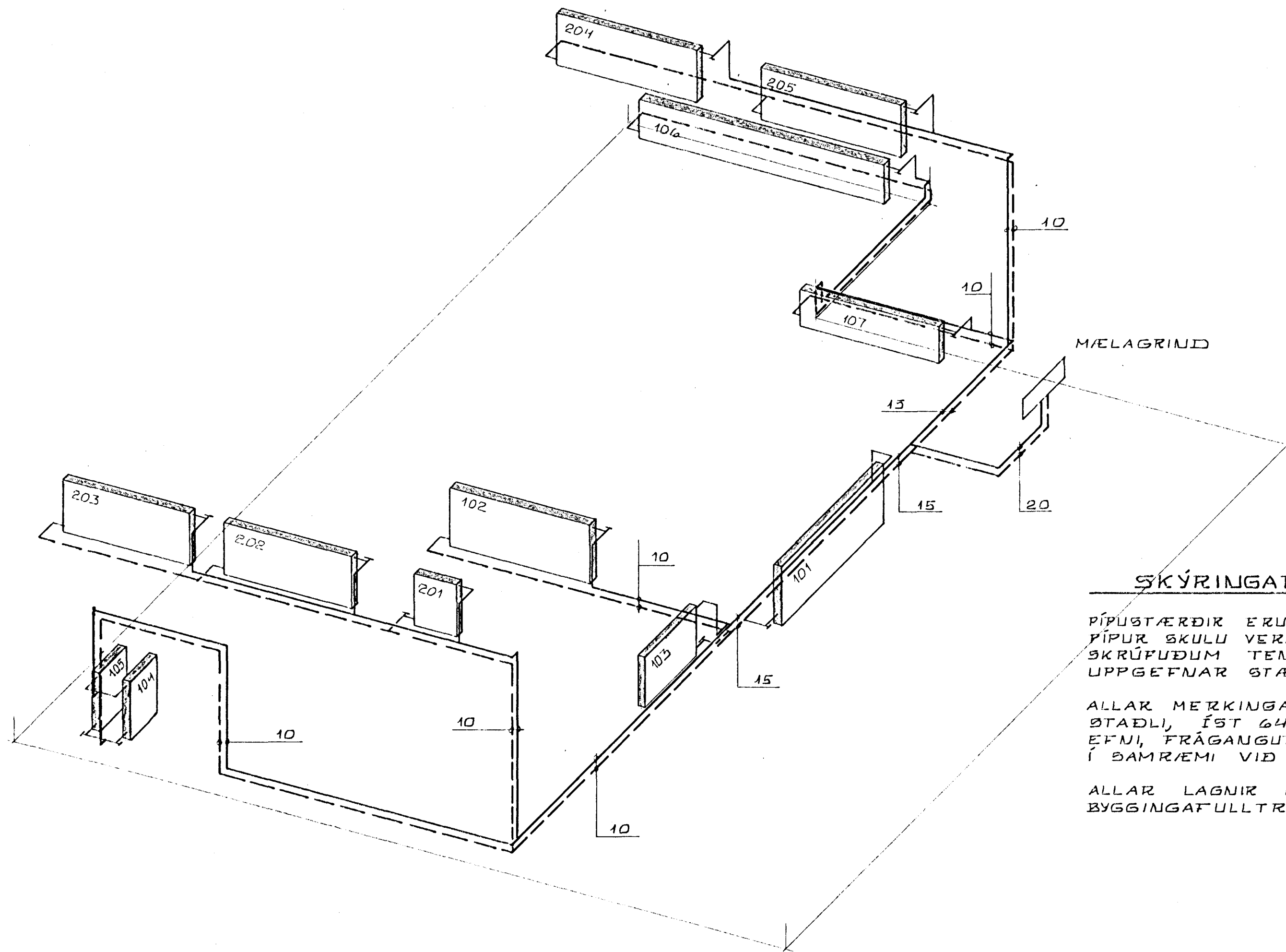
RÚMMYND HITALAGNA 1:50
