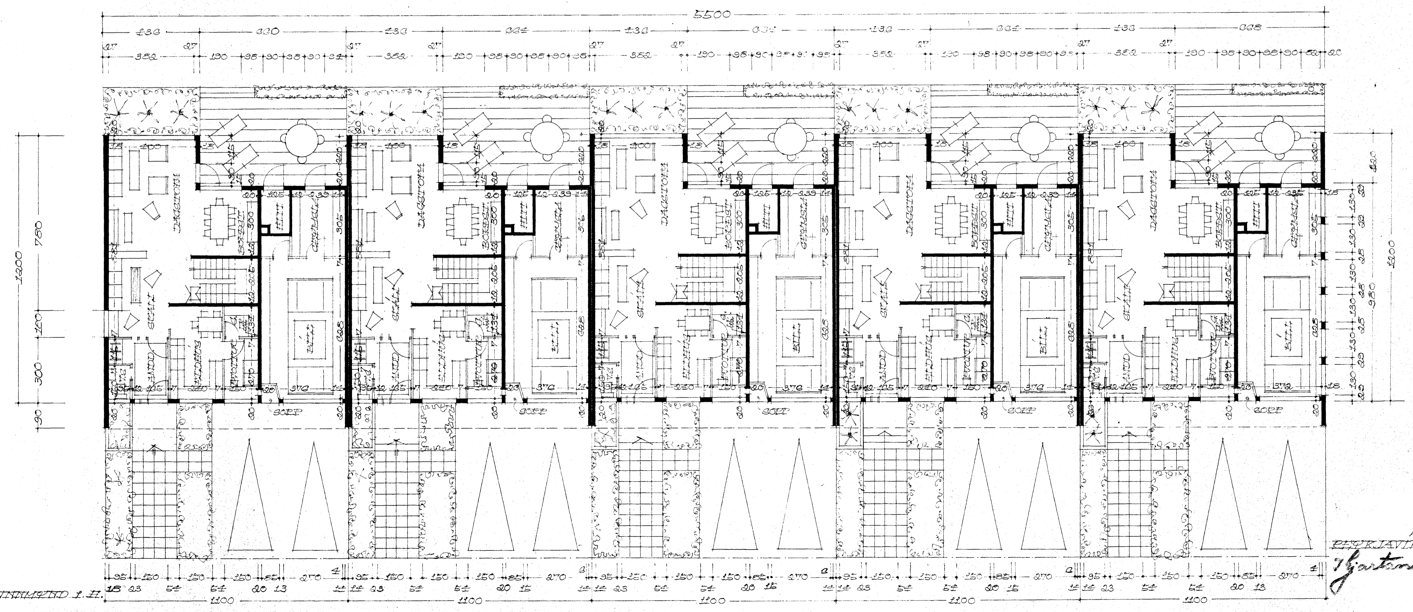
GRUNNHAUÐ 2. HAÐ
