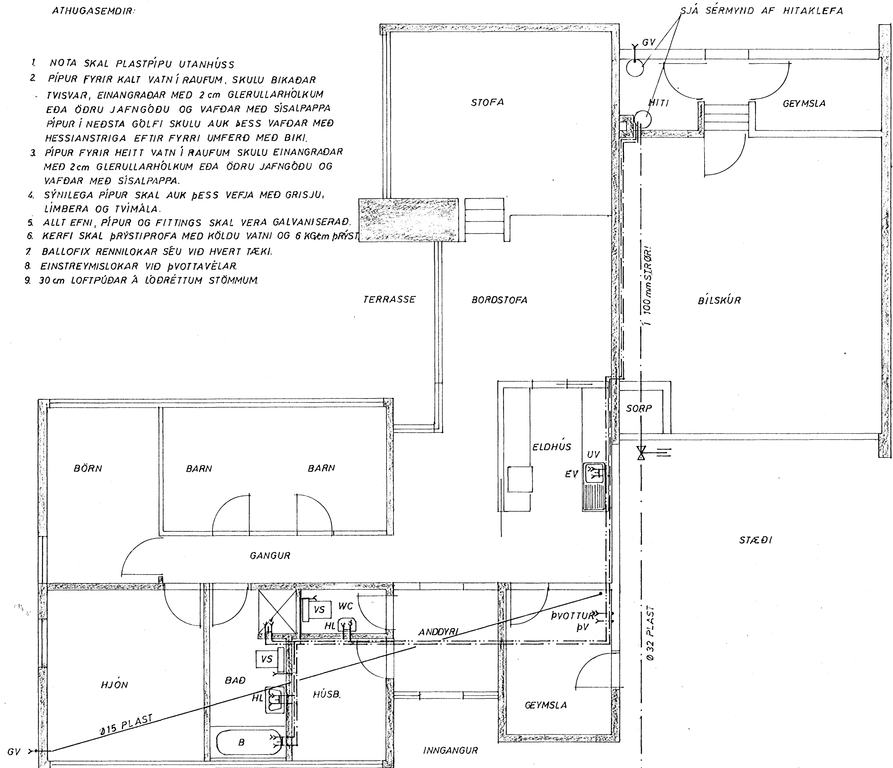
GRUNNMYND 1:50
