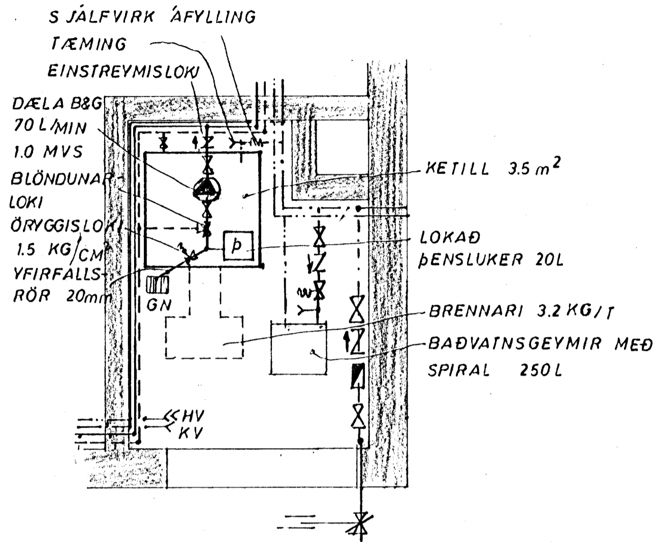
GRUNNMYND HITAKLEFA 1:20
