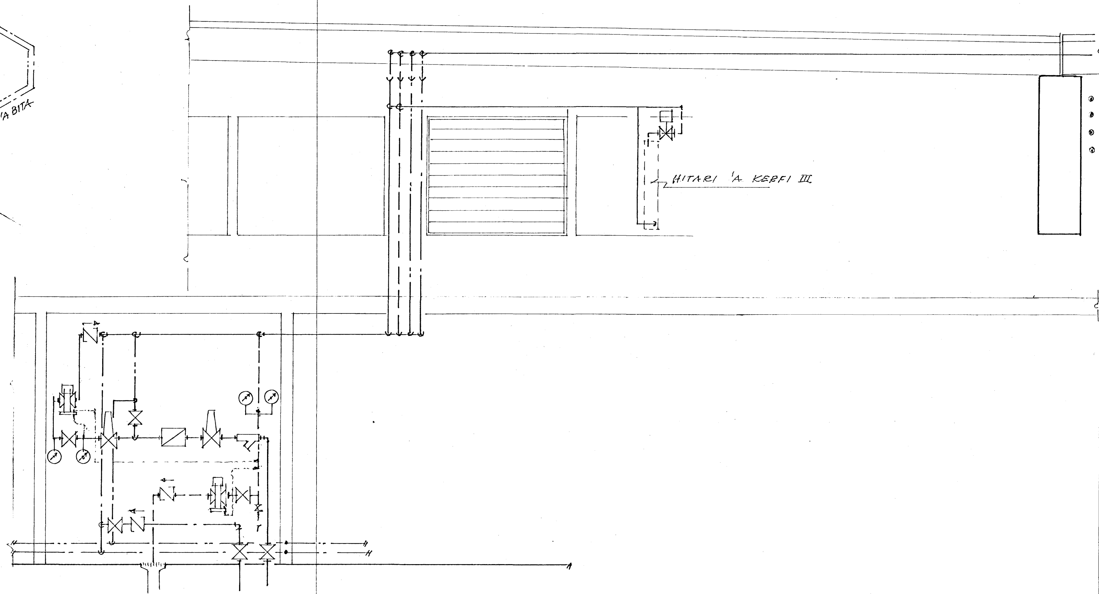
VATNSKLEFI - MÆLAGRINDUR 1:20
