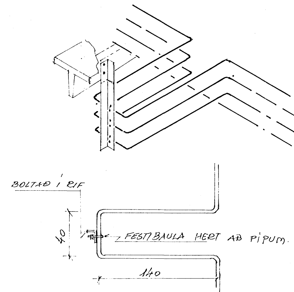
FENSLUBEYGGJUR 'A' MIÐSÚLU ~ 1:20
