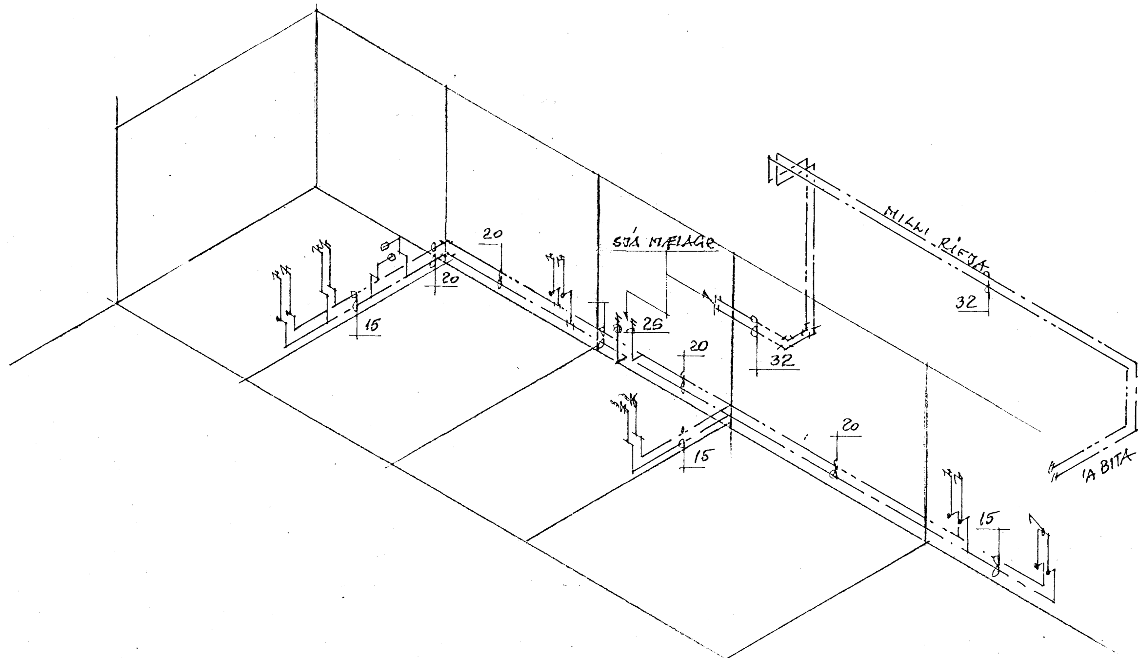
VATNSLÖGN - RÚMMYND - AUSTURENDI ~ 1:50
