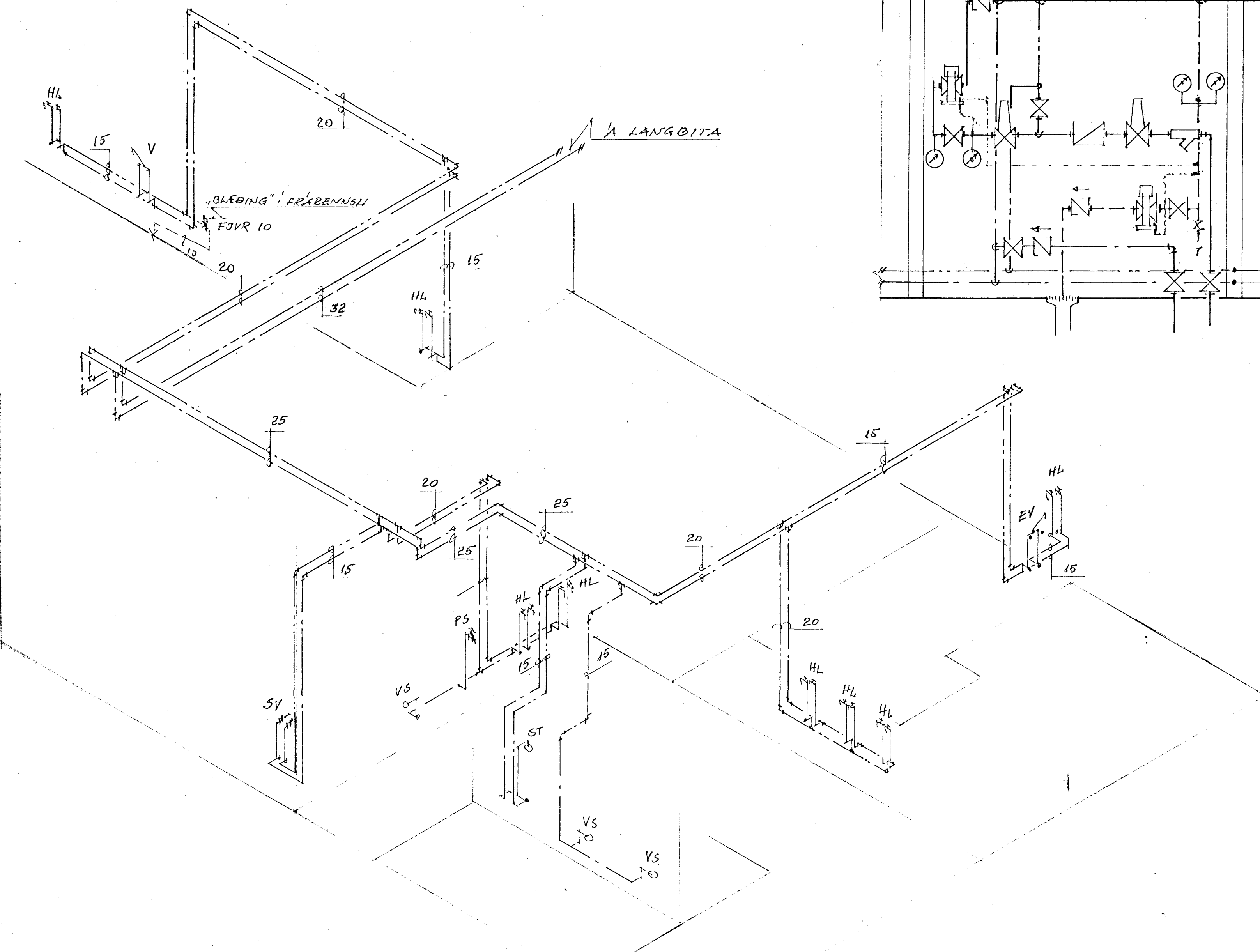
VATNSLÖGN - RÚMMYND - VESTURENDI ~ 1:50
