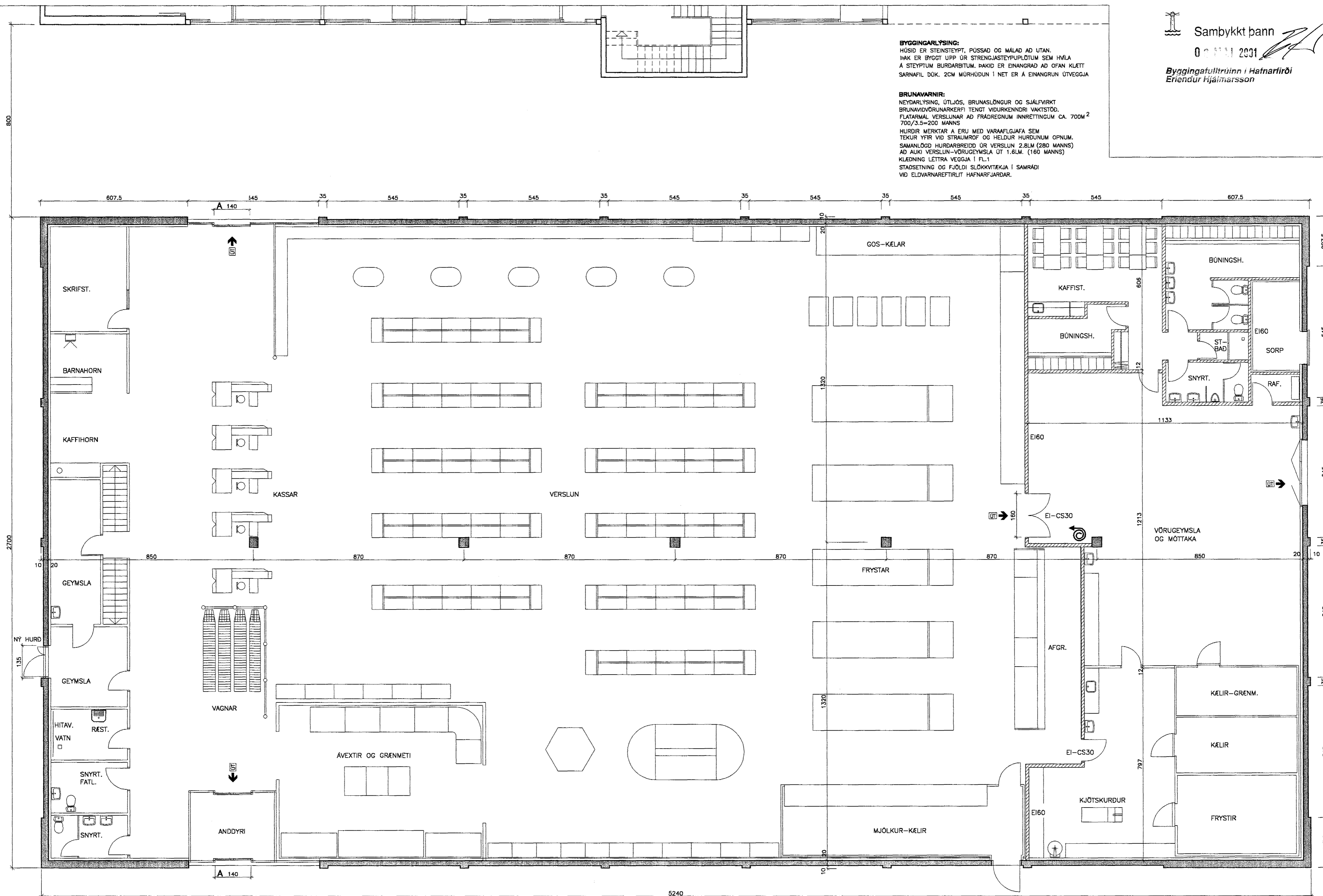
GRUNNMYND 1.HÆÐ
