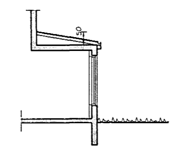
Snið í gegnum þak yfir sperru mkv. 1:100
