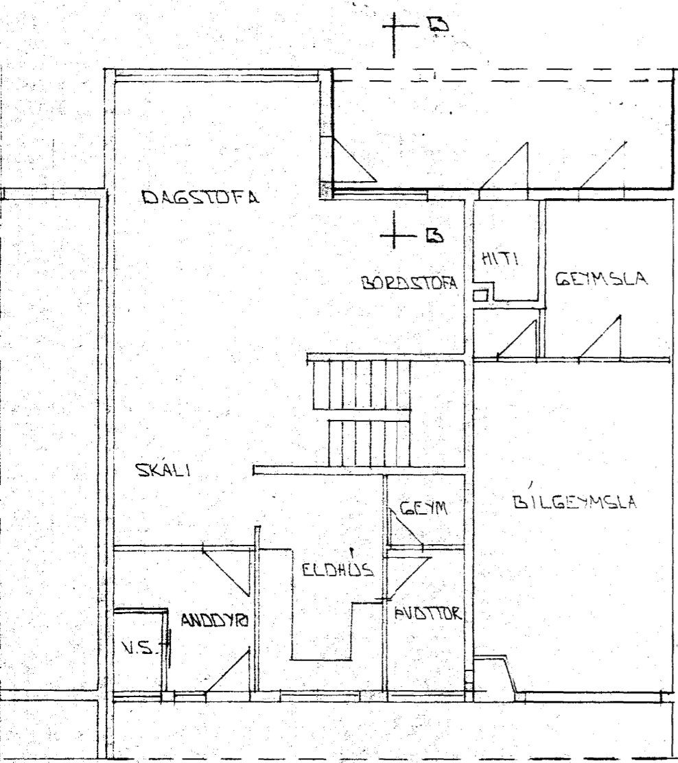
GRUNNMÝND 1. HÆÐ 1:100
