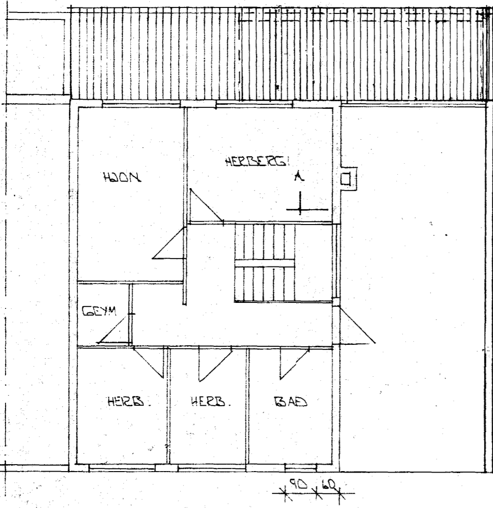
GRUNNMÝND 2. HÆÐ 1:100
