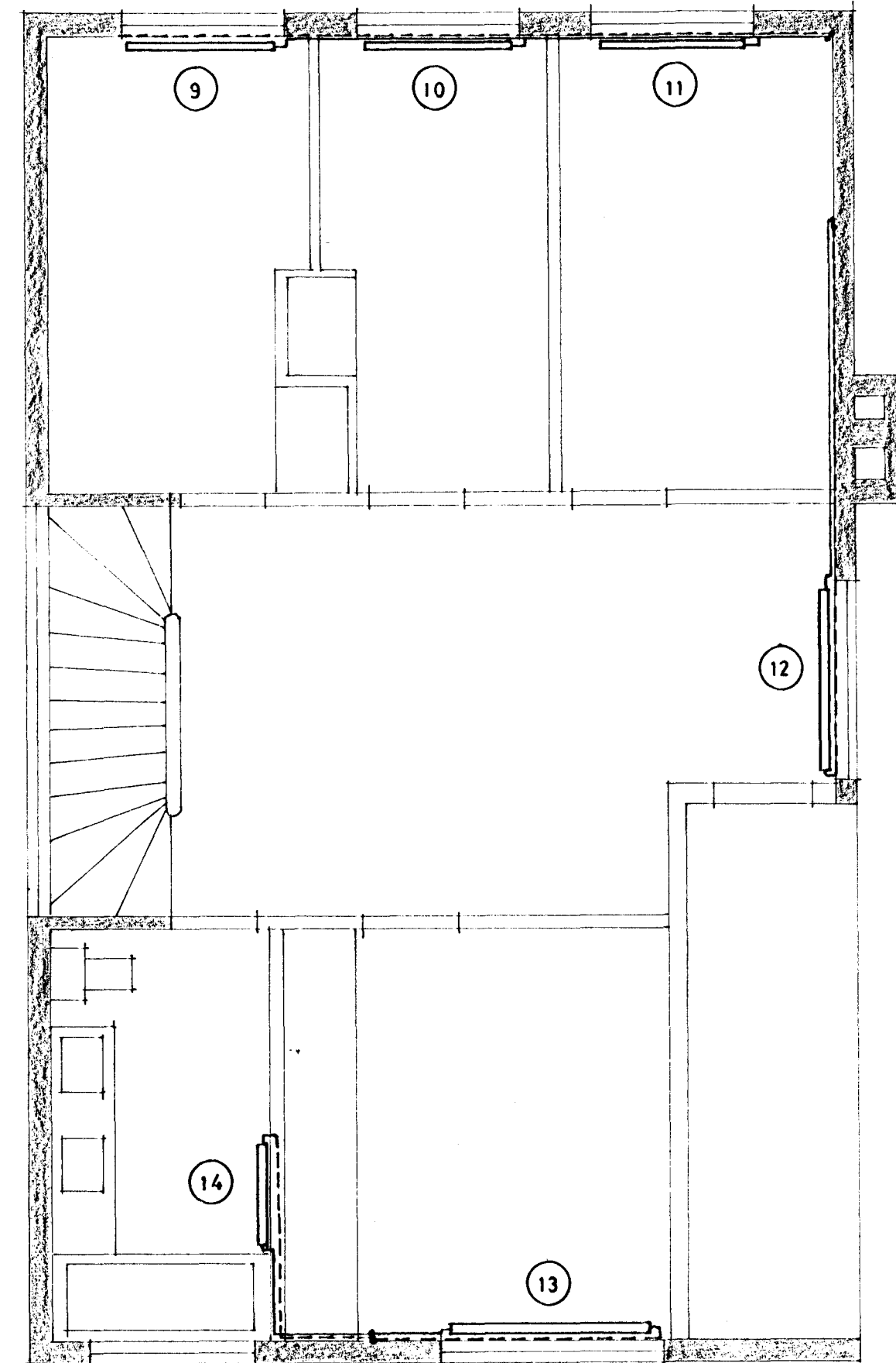
GRUNNMYND 2. HÆÐ
