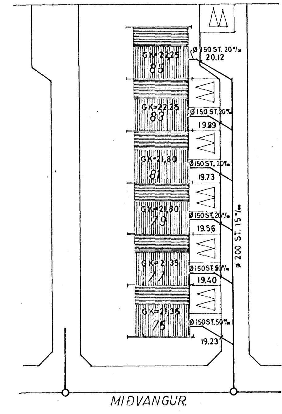
AFSTÖÐUMYND 1:500
