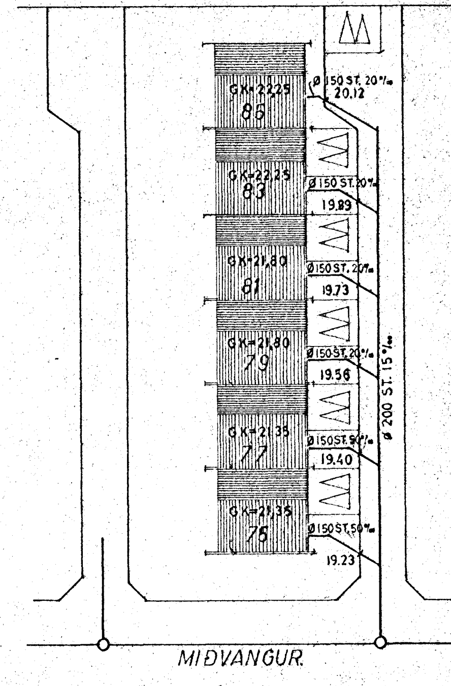
AFSTÖÐUMYND 1:500
