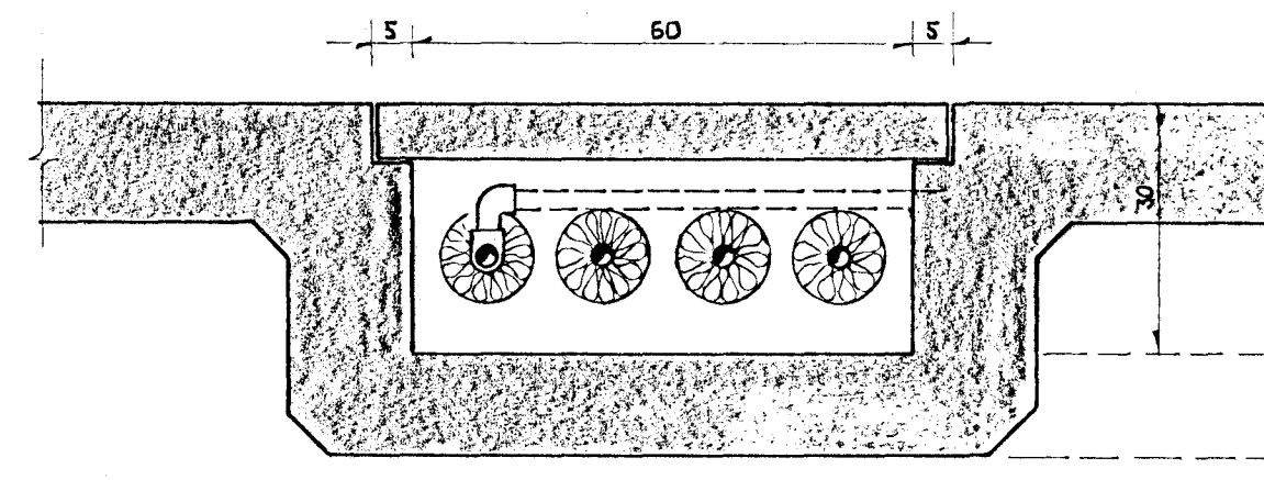
STOKKUR A 1:10
