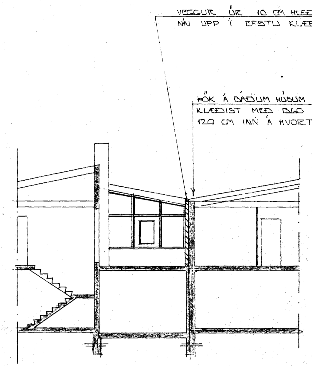
SNID A-A 1:100
