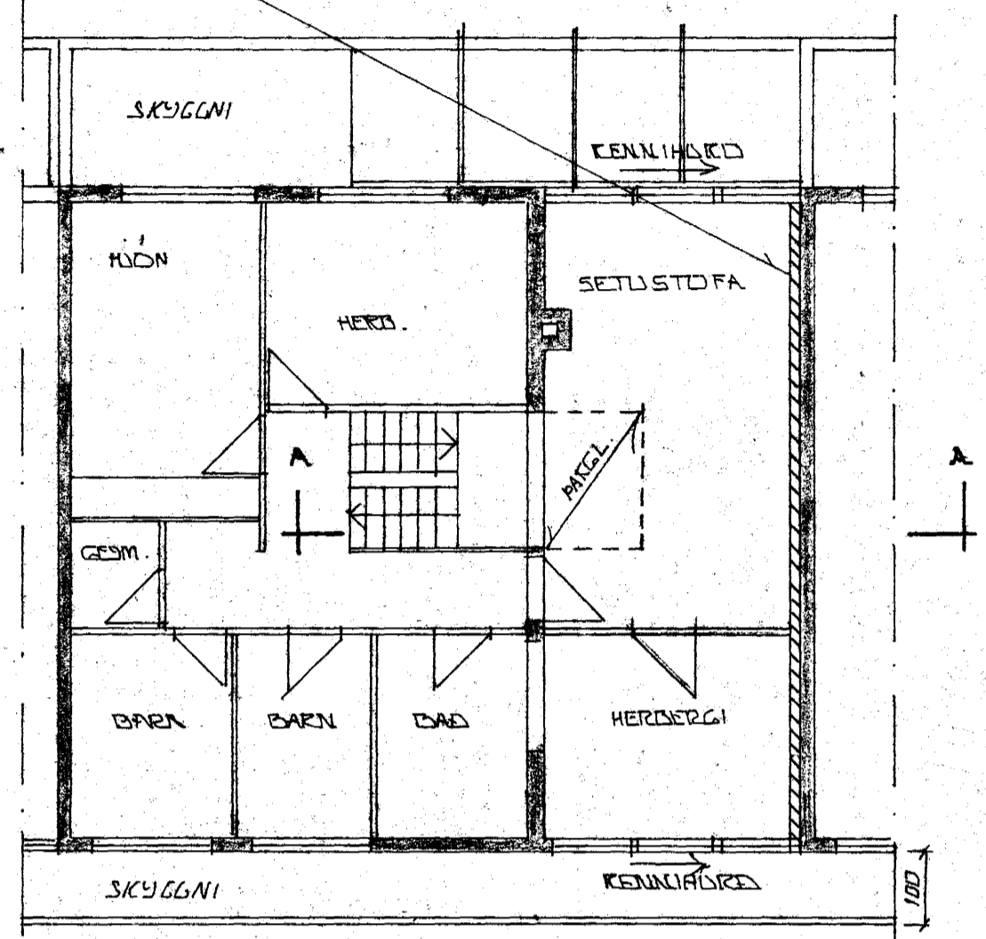
FLORNAÐMYND 1:100
