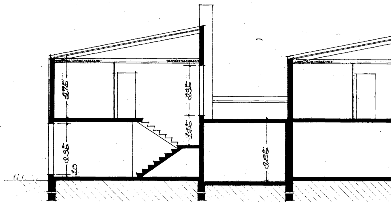
SKURÐUR B-B
