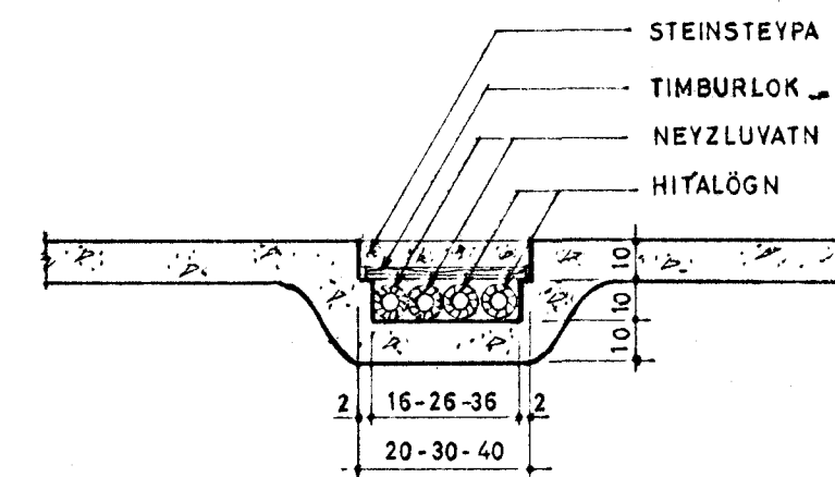
GÓLFRAUF M=1:20
