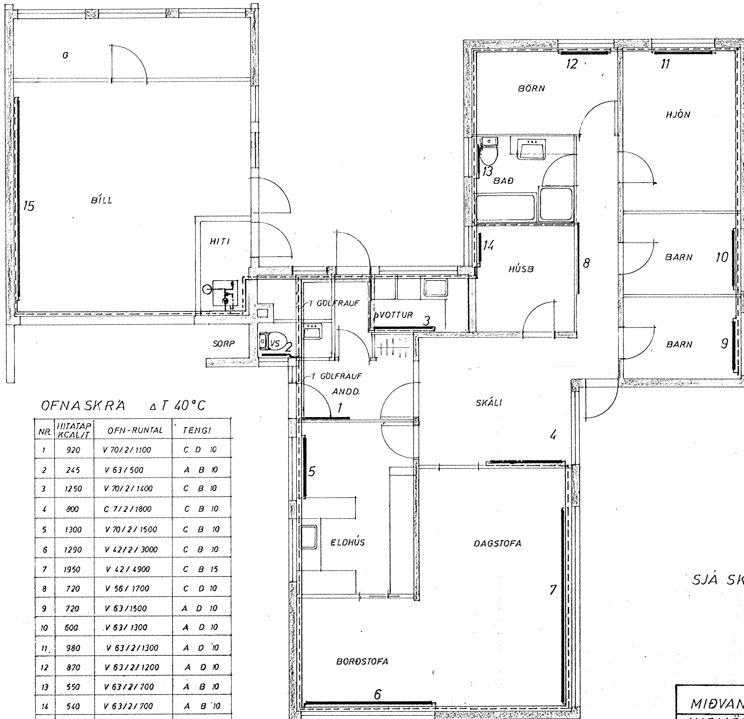
GRUNNMYND 1:50
