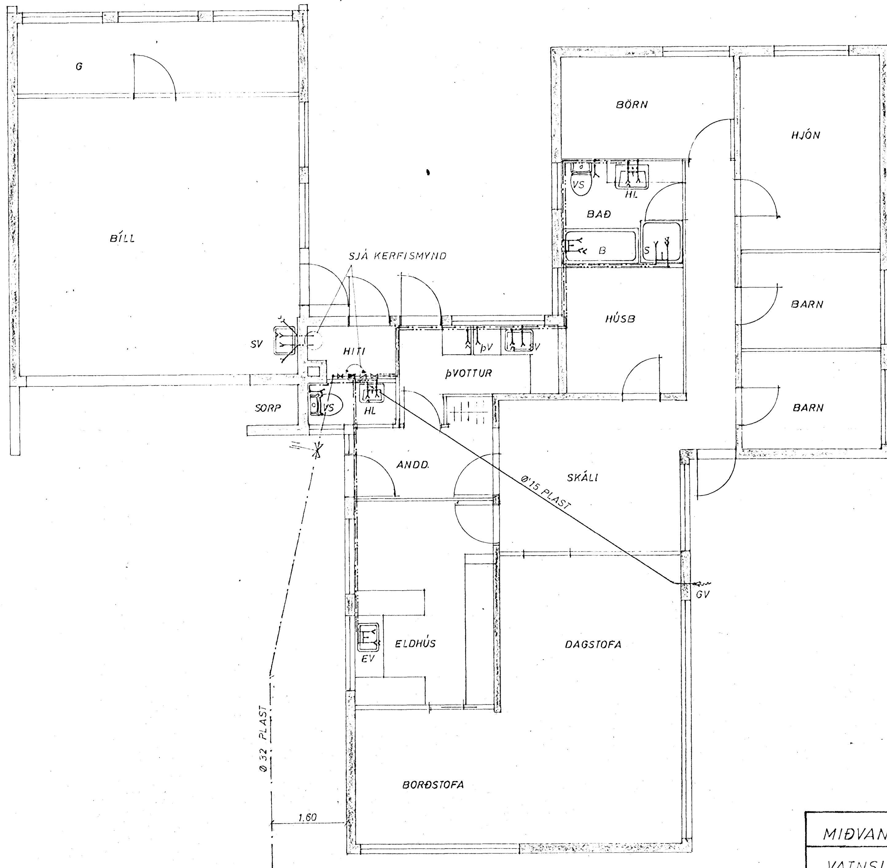
GRUNNMYND 1:50
