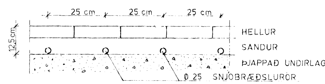
SNJÓBRÆÐSLURÖR ÞVERSNIÐ Í STÉTT
