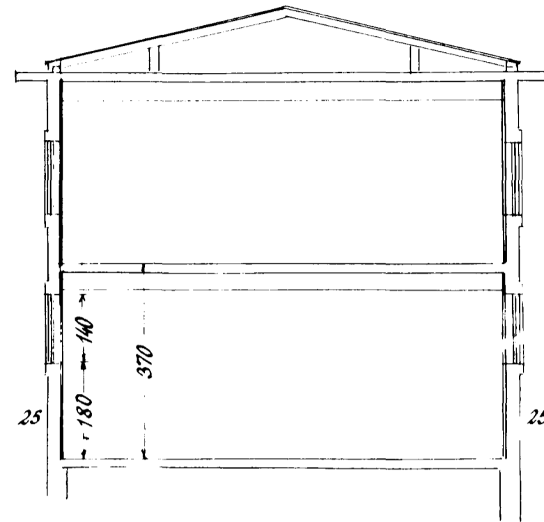
Þverskurður
