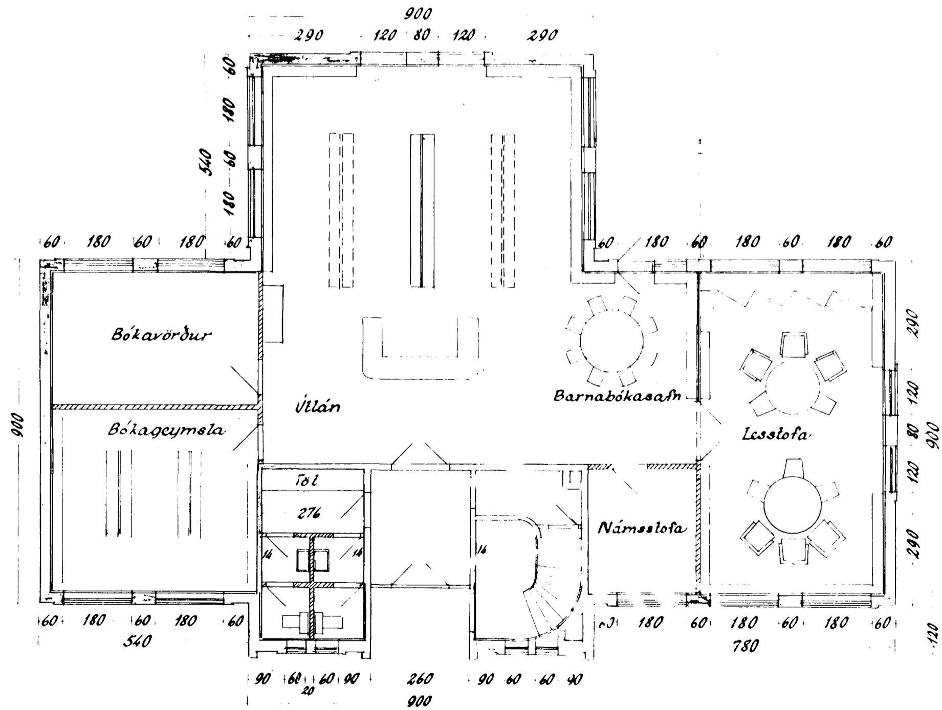
Grunnmynd 1. hæðar
