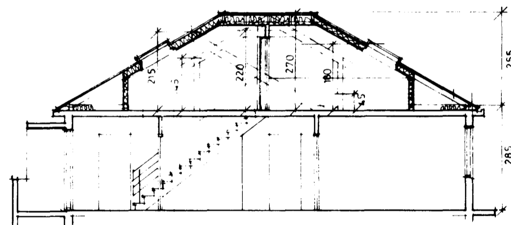
SNIÐ A-A
