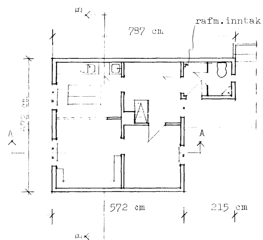
Grunnmynd 1. hæð
