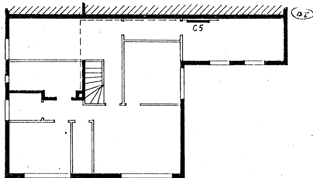
GRUNNMYND KJALLARA
