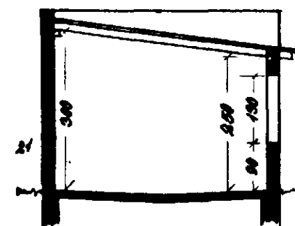
Þverskurður
