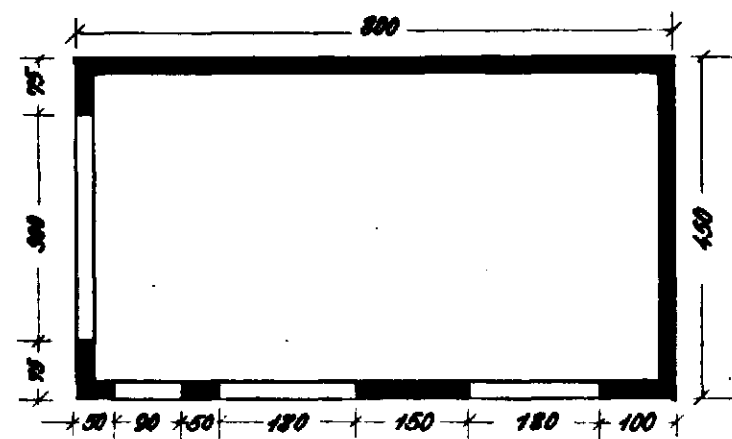
Grunnamynd
