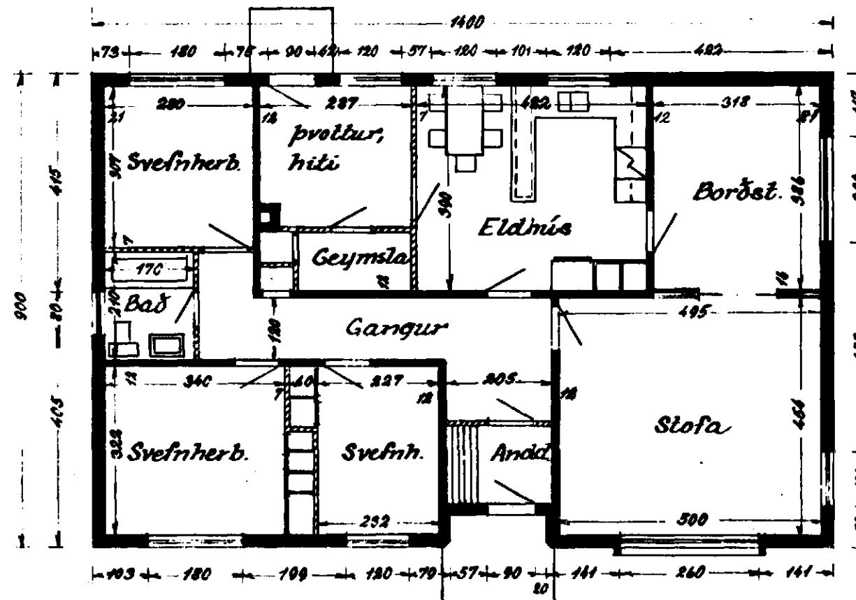
Grunnmynd
