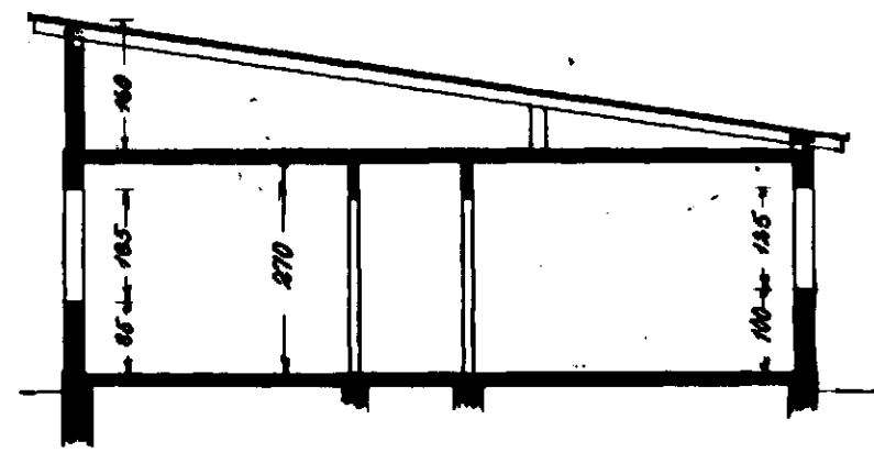
Þverokurður
