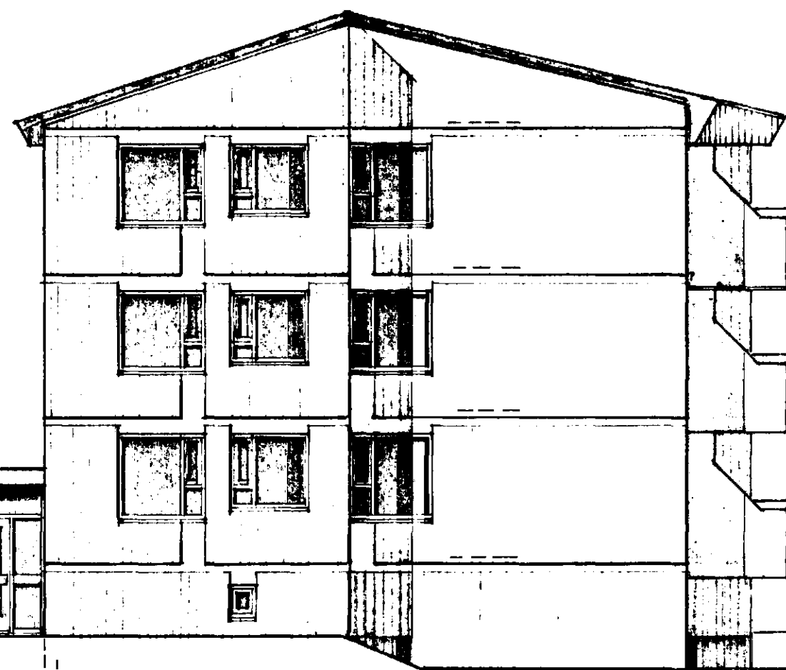
NORÐVESTURHLIÐ
