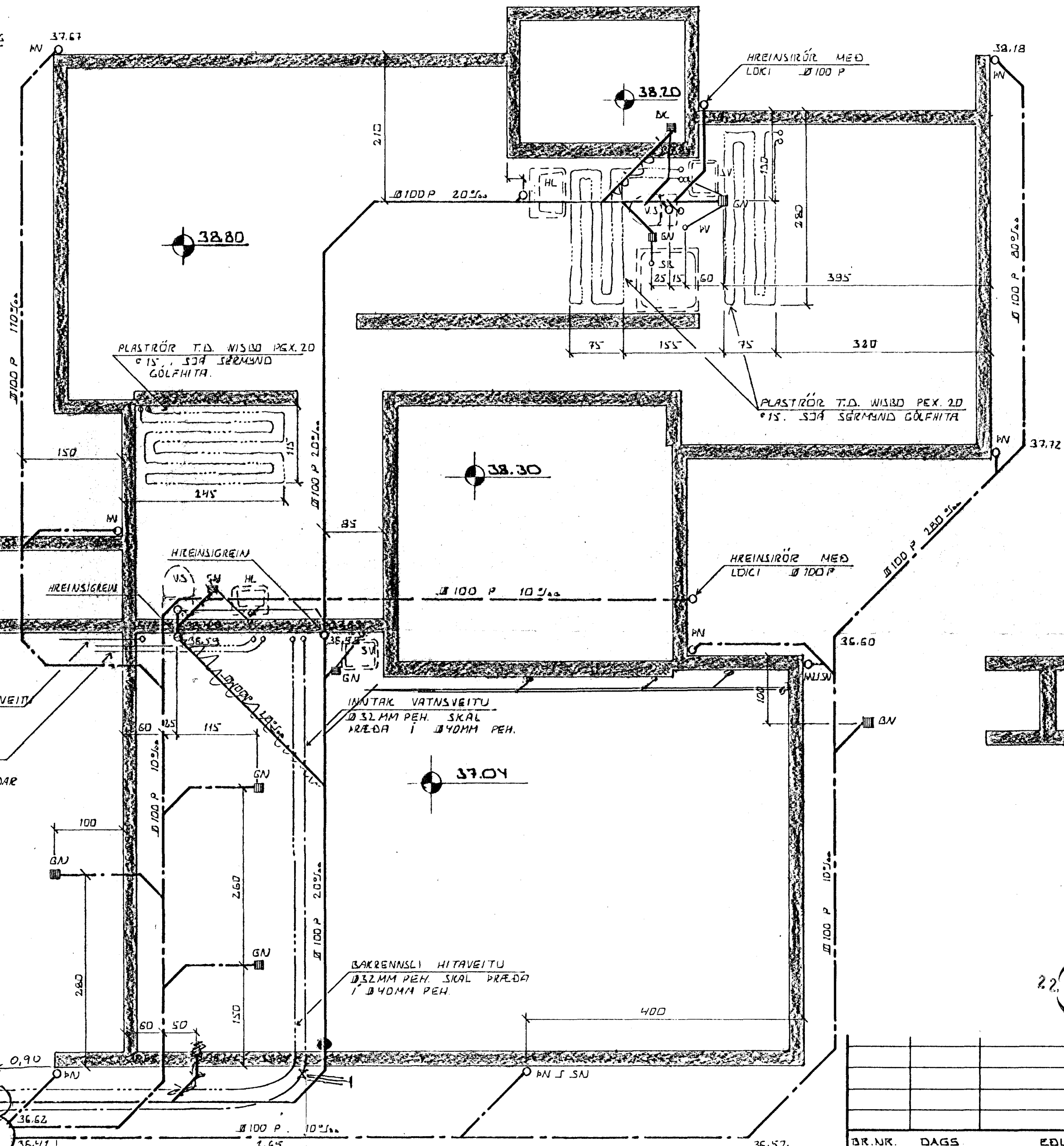
GRUNNMÝND 1:50
