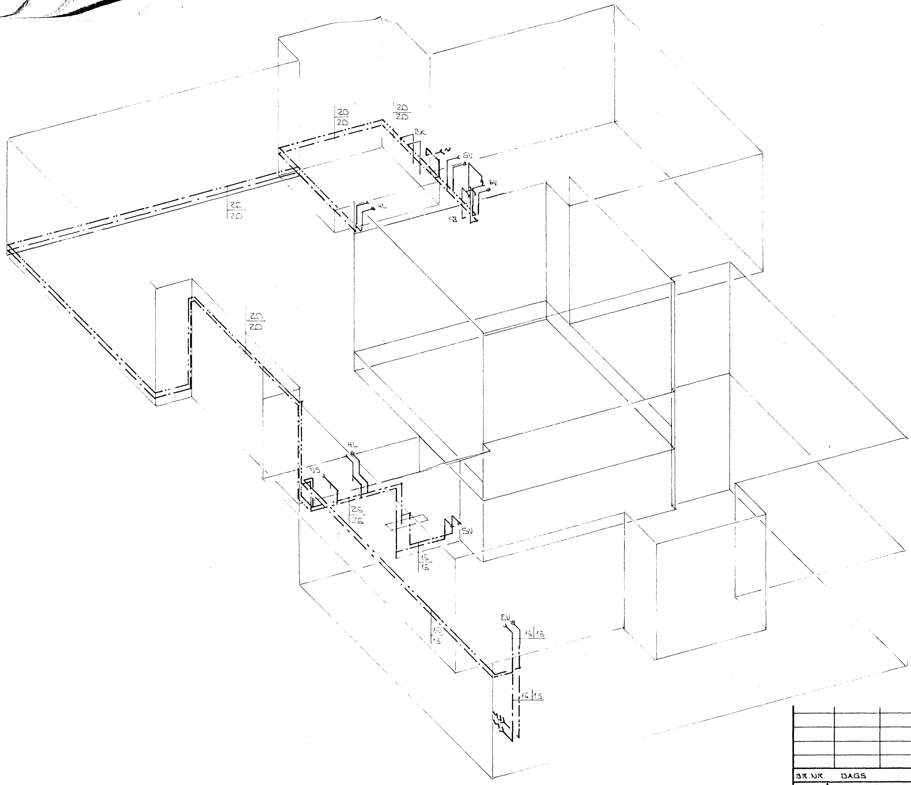
RÚMMYND VATNSLAGNA 1:50
