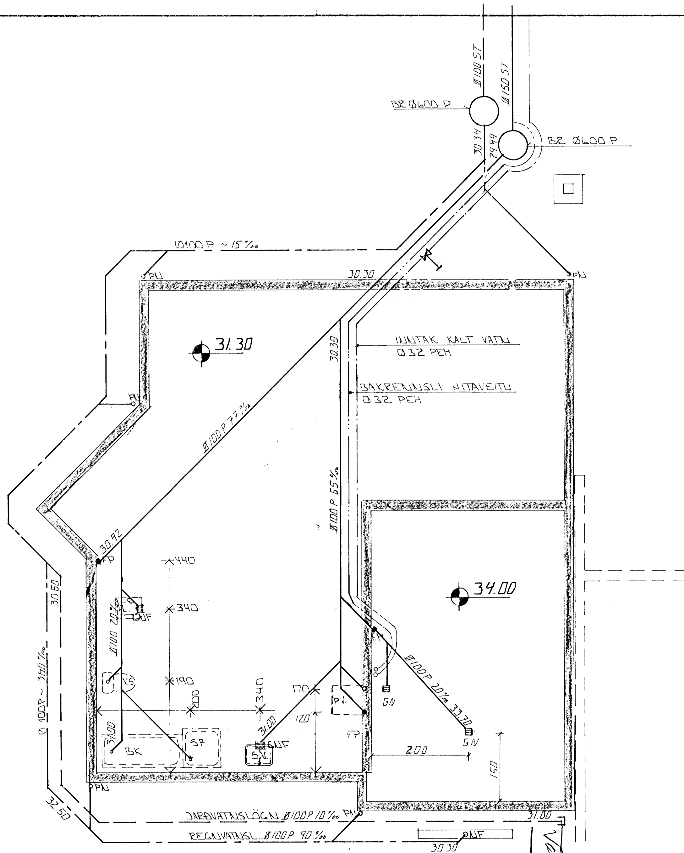
GRUNNMYND • 1 : 50
