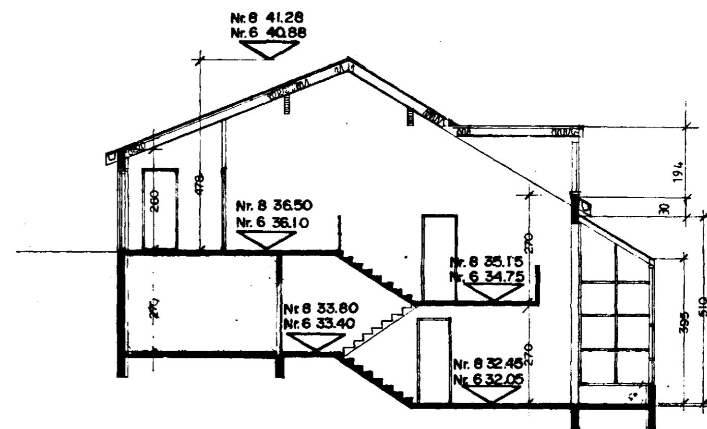
SKURÐUR A-A
