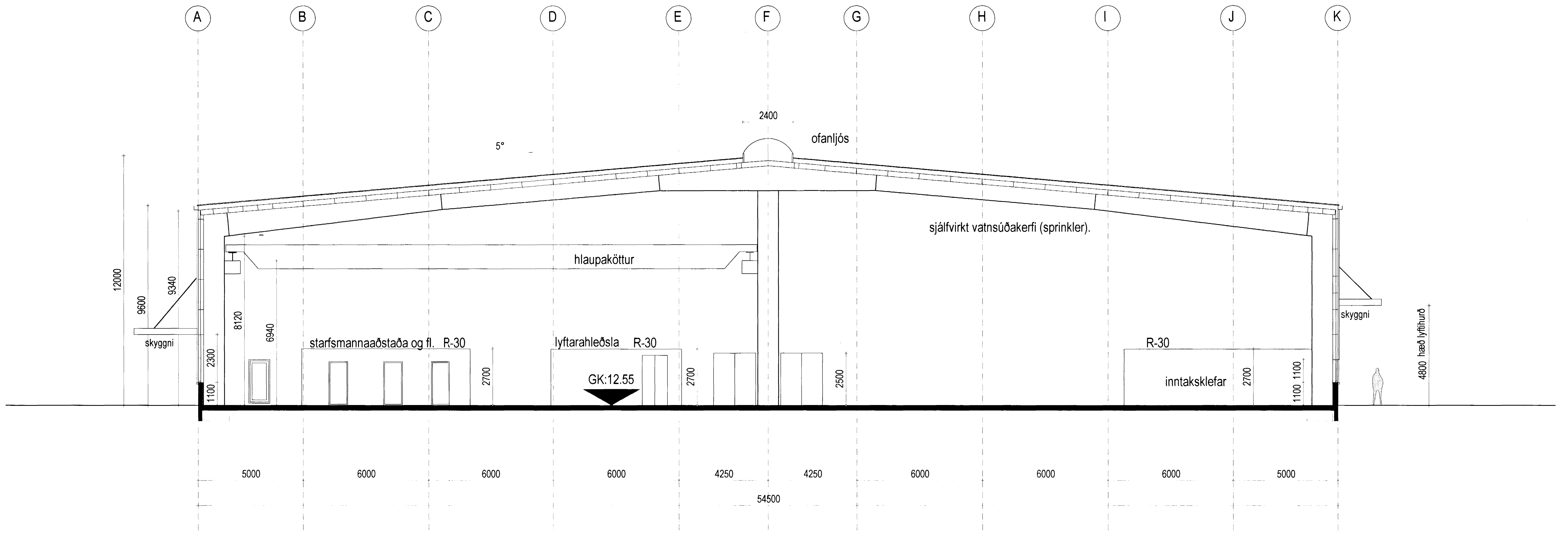
SNEIDING A-A
