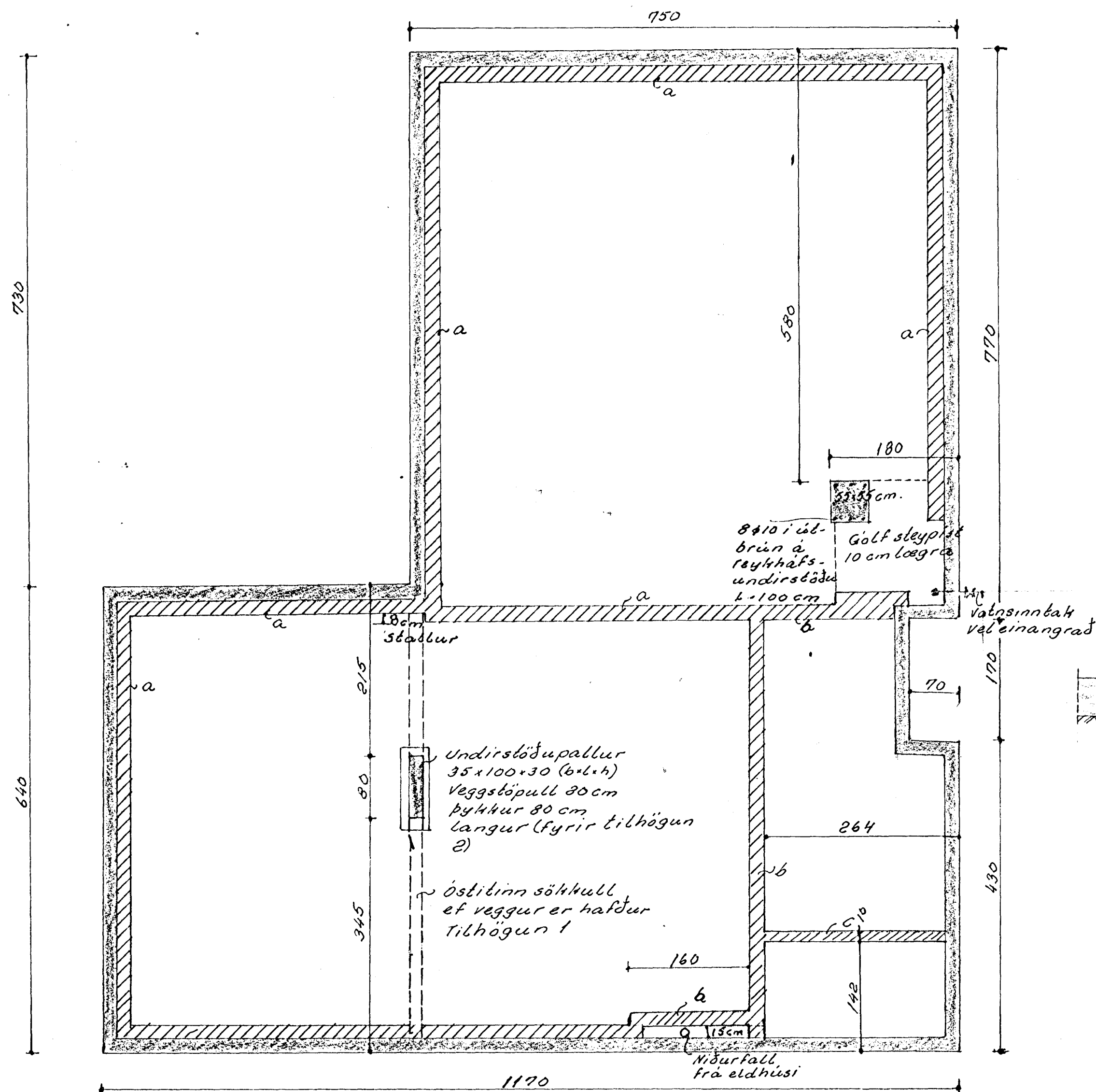
Grunnmynd 1:50
