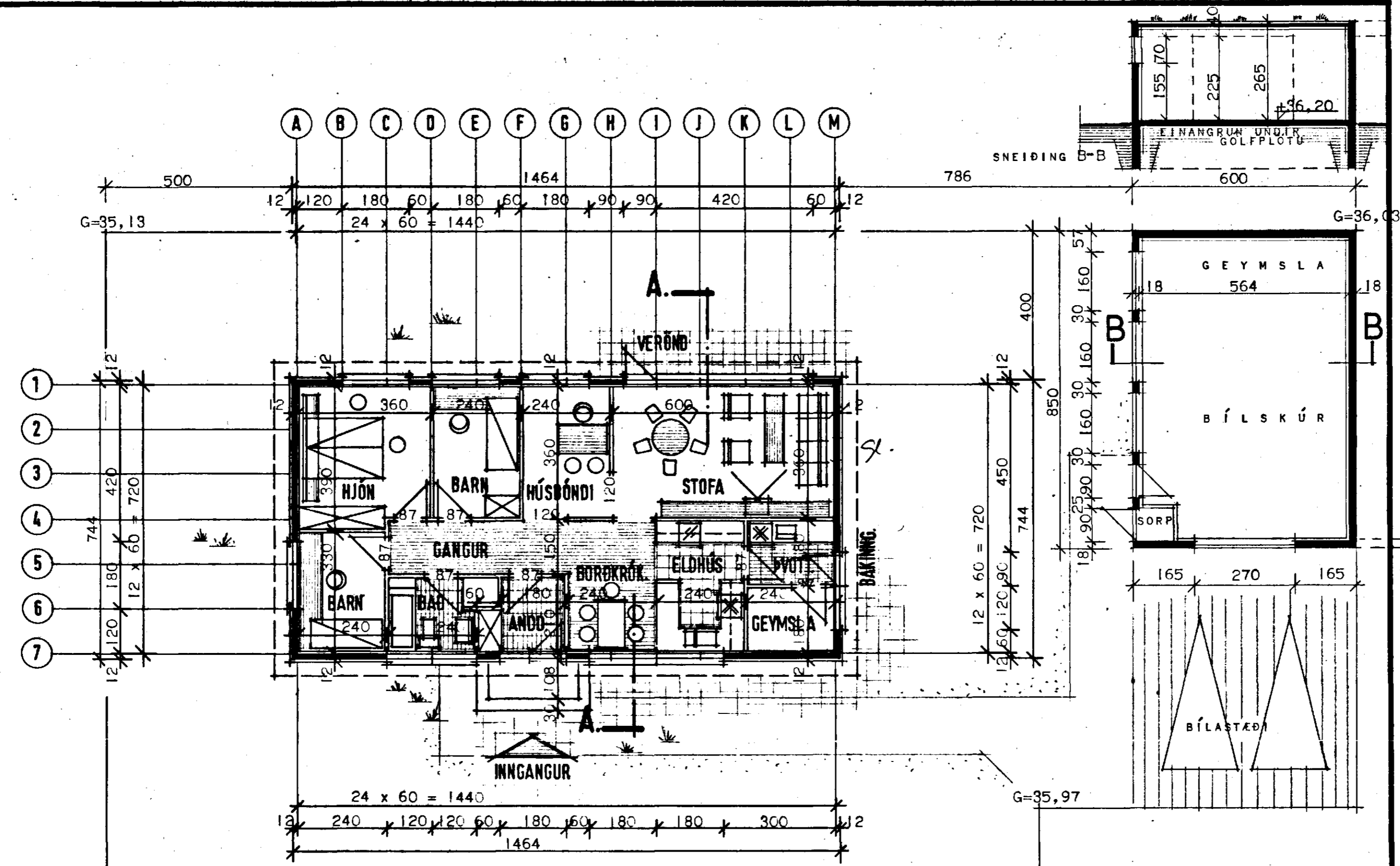
GRUNNMYND.
