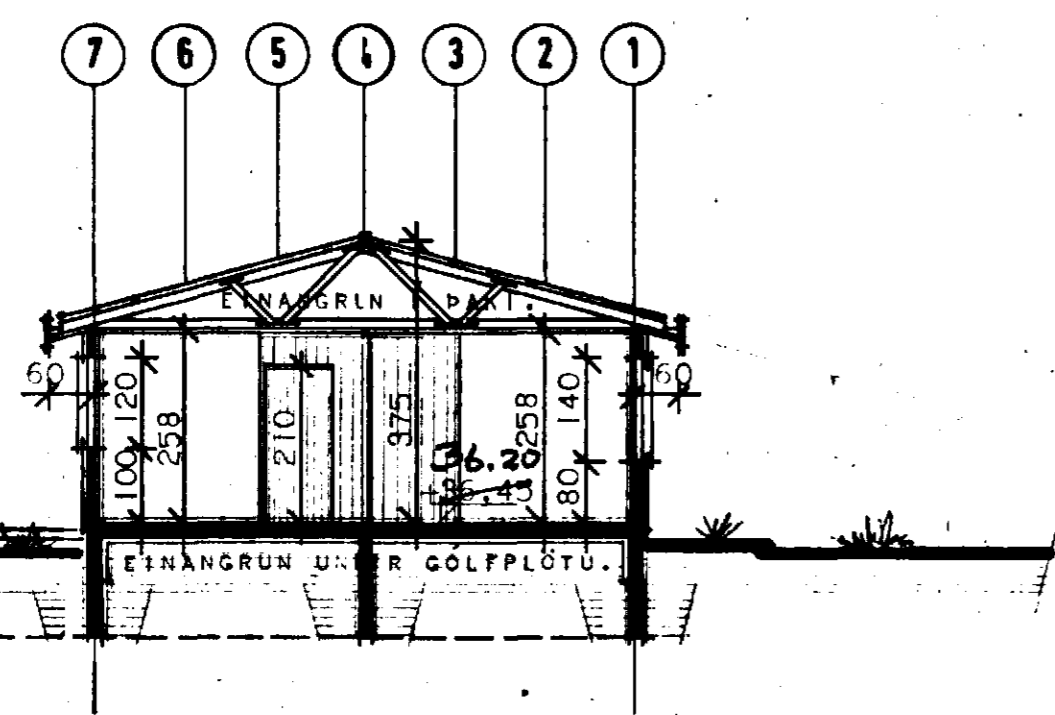
ÞVERSNEIÐING A-A.
