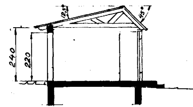
Snið A-A
