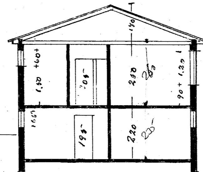
Þverskurður
