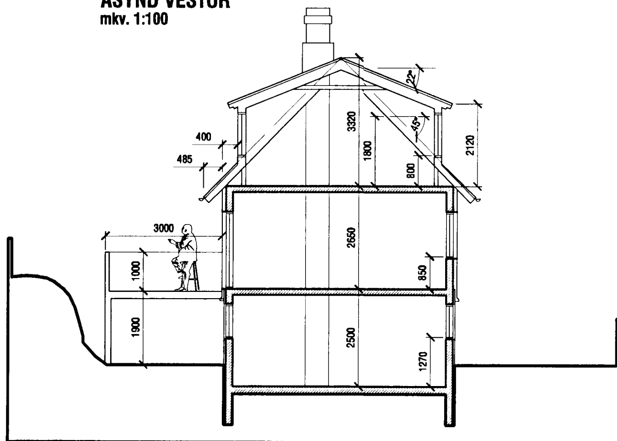
SNEIÐING A-A mkv. 1:100
