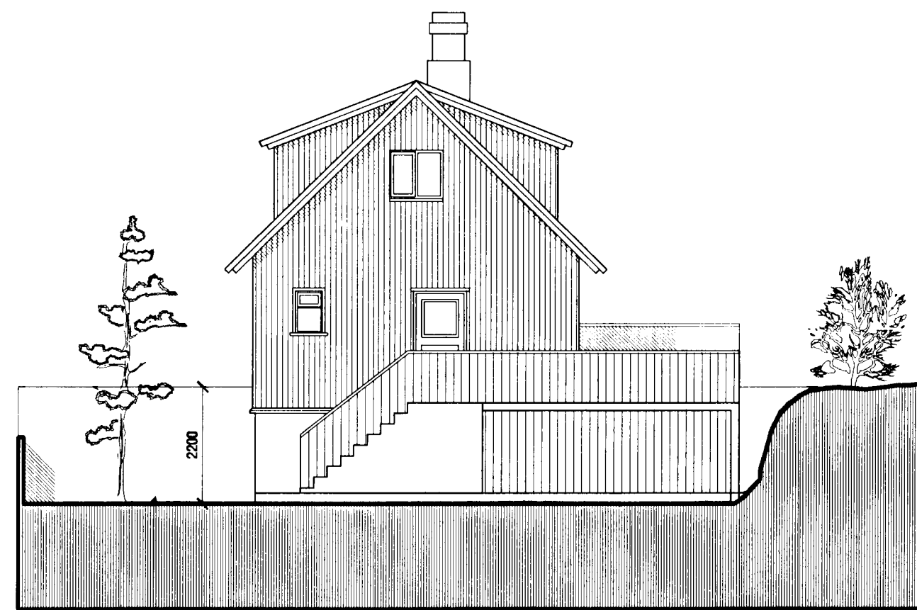
ÁSÝND SUÐUR mkv. 1:100
