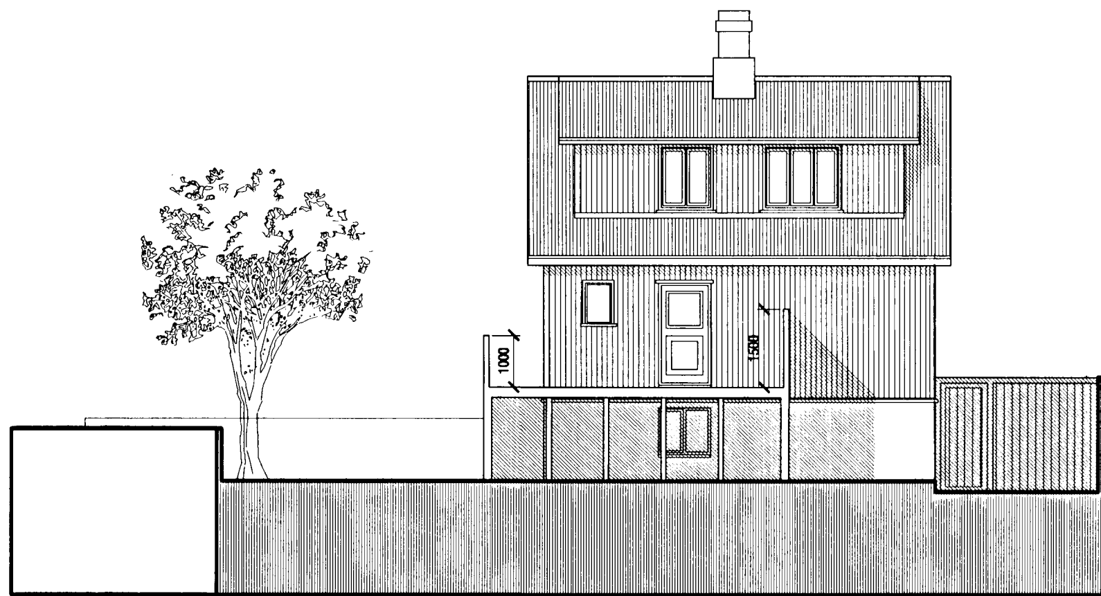
ÁSÝND AUSTUR mkv. 1:100
