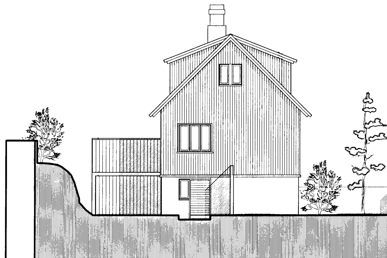
ÁSÝND NORÐUR mkv. 1:100
