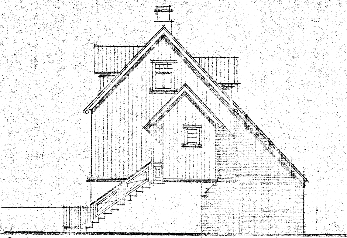
AUSTUR M. 1:100
