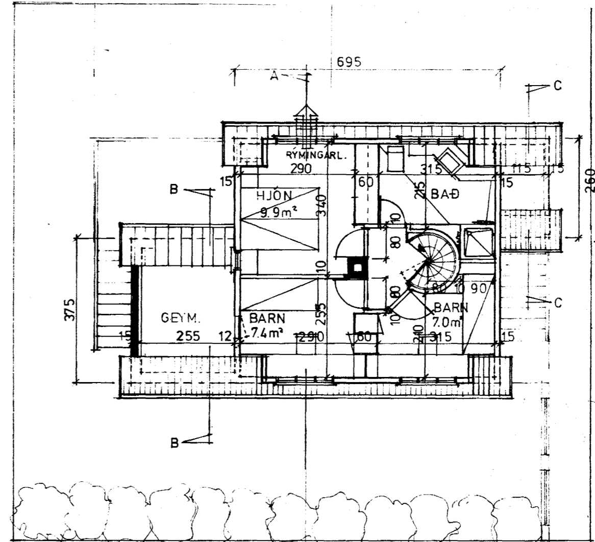
RÍS BRUTTÓ: 55.4 M 2
