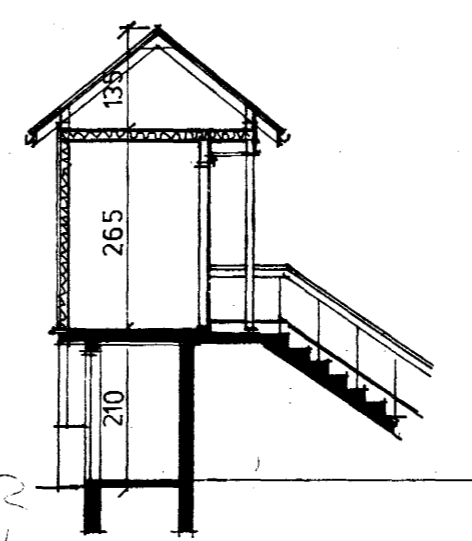
SNIÐ C - C
