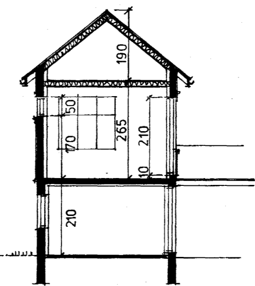
SNIÐ B - B
