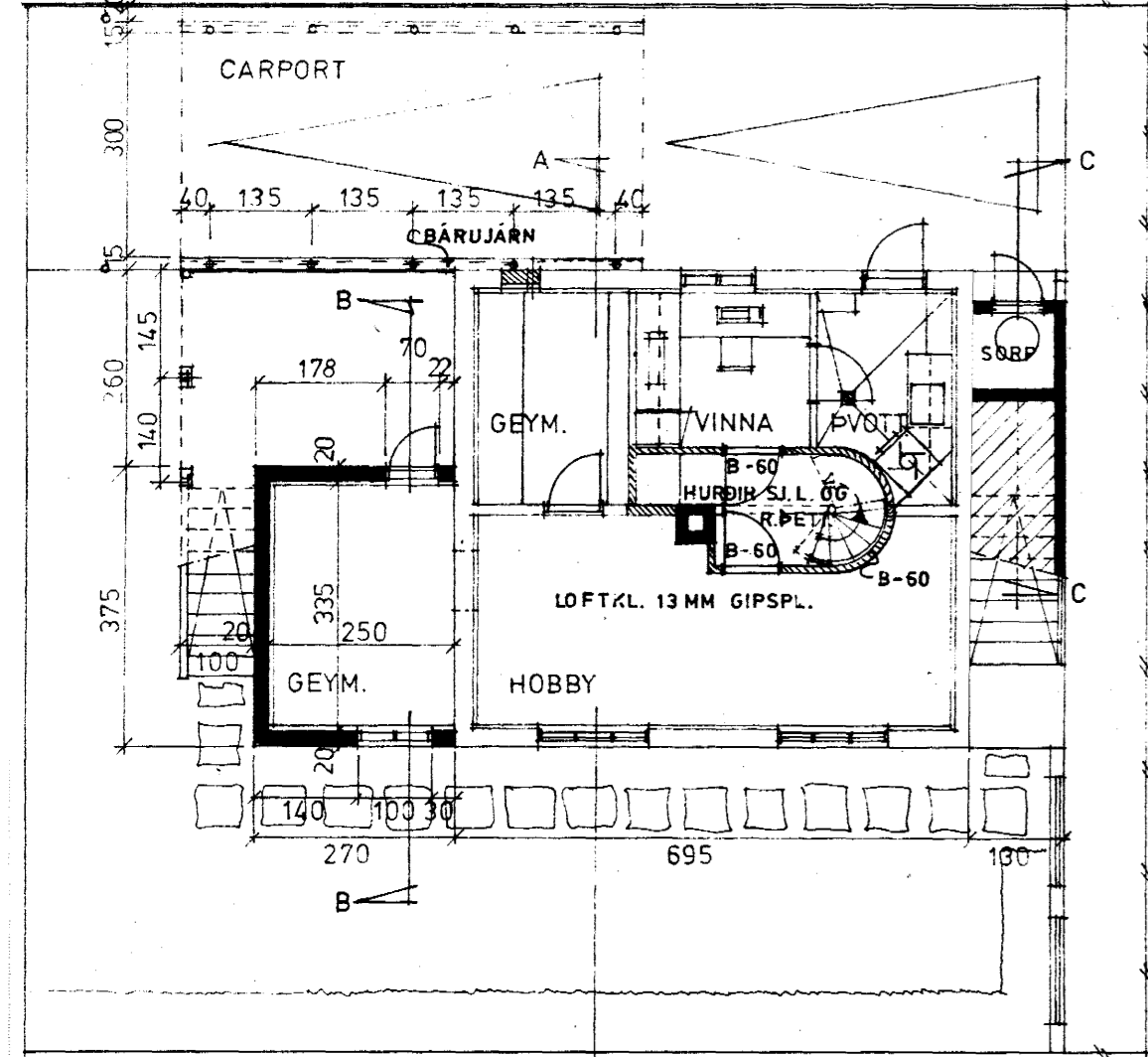
JARDHÆÐ BRUTTÓ: 54.2 M 2
