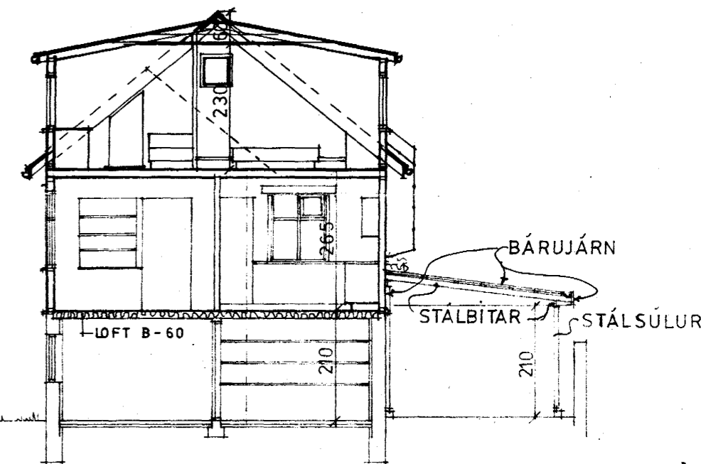
SNIÐ A - A
