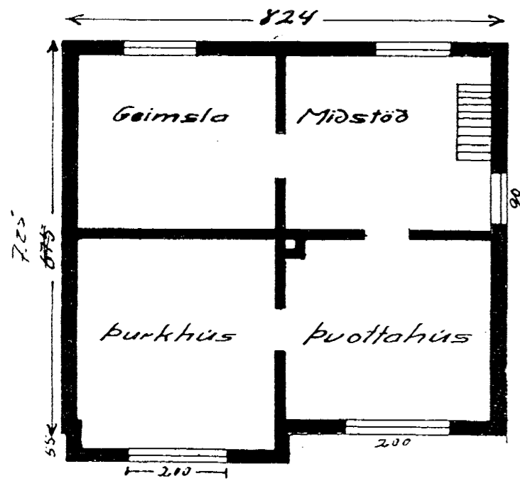
Kjallari
