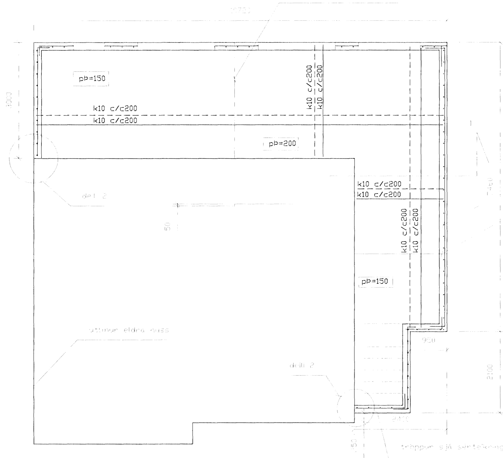
Grannmynda kjallara 1/80
