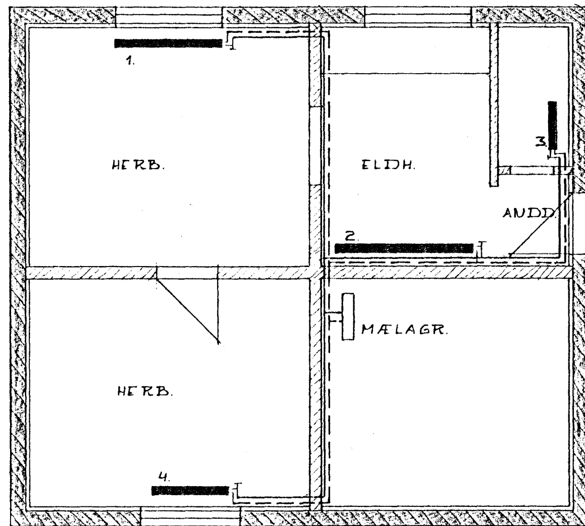
GRUNNMYND JARÐHÆÐAR ~ 1:50
